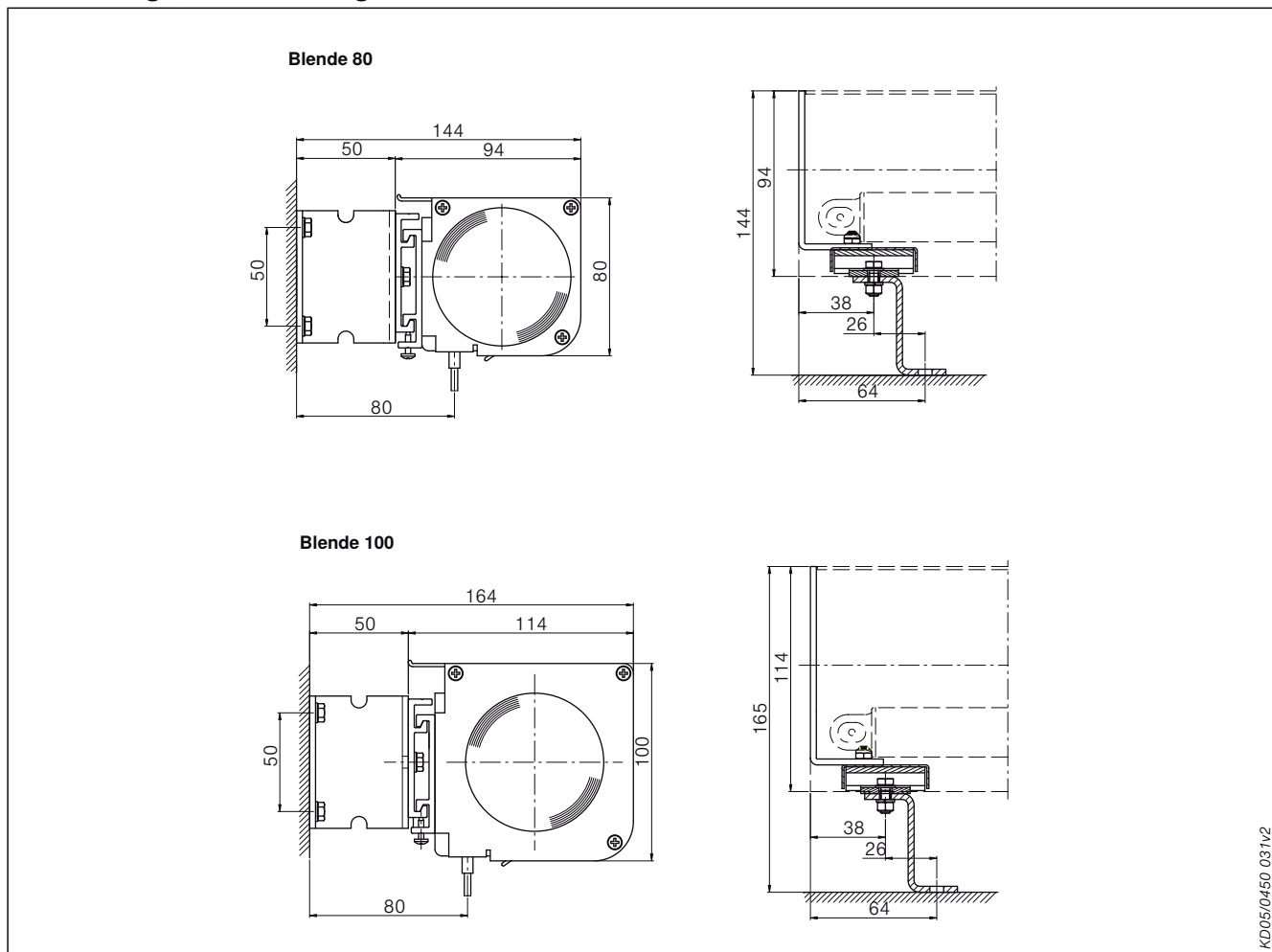
Abb. 119: Maßblatt
