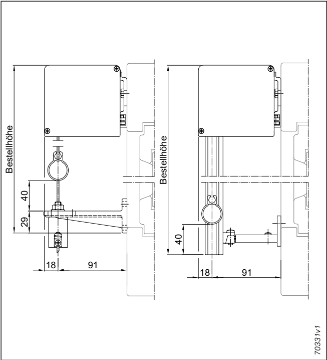
Abb. 36: Senkrecht-Markise 490 Wandmontage
