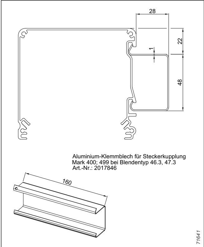
Abb. 288: Klemmblech für Steckerkuplung, Senkrecht-Markisen
