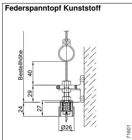
Abb. 69: Federspanntopf Kunststoff
