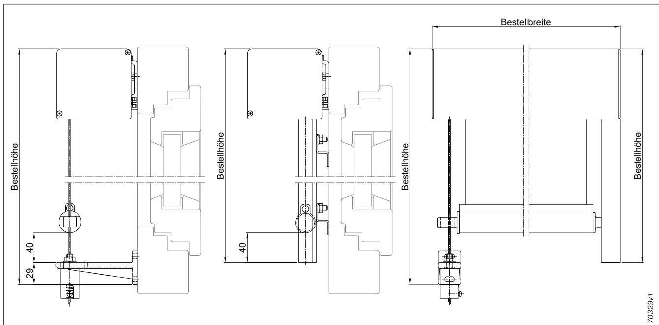
Abb. 28: Maßanleitung
