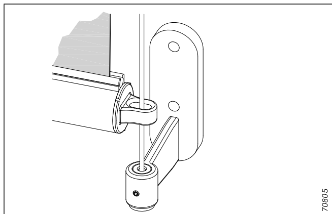
Abb. 206: Spannseil
