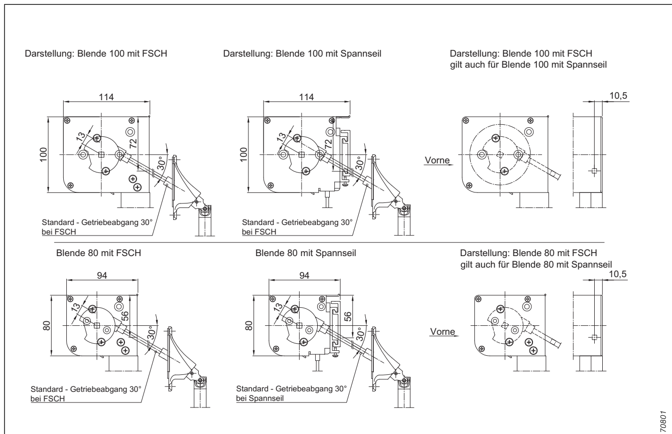
Abb. 124: Getriebeabgang 30°
