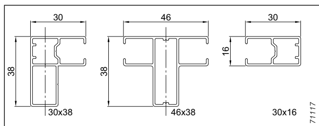
Abb. 107: Führungsschienen
