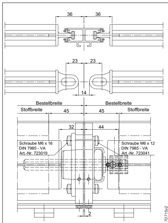
Abb. 80: Kupplungsmöglichkeiten und Reihenanlagen bei Typ 499: Kupplung Einzelblende Standard
