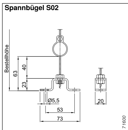
Abb. 31: Spannbügel S02
