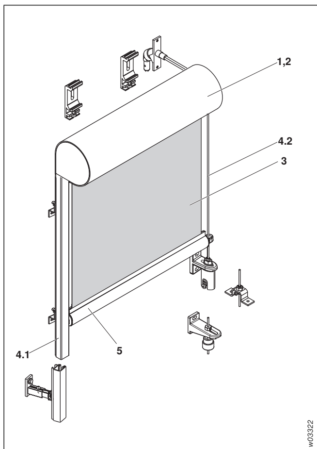
Abb. 62: Senkrecht-Markise 499
