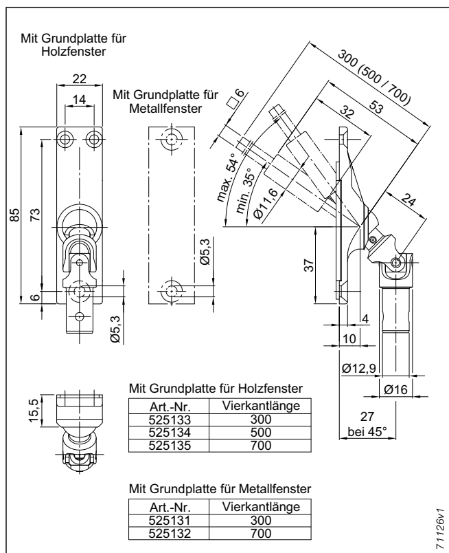
Abb. 233: Gelenkplatte 35°–54°
