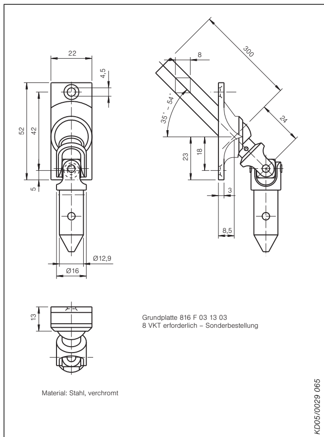
Abb. 194: Gelenkplatte 35°–54°
