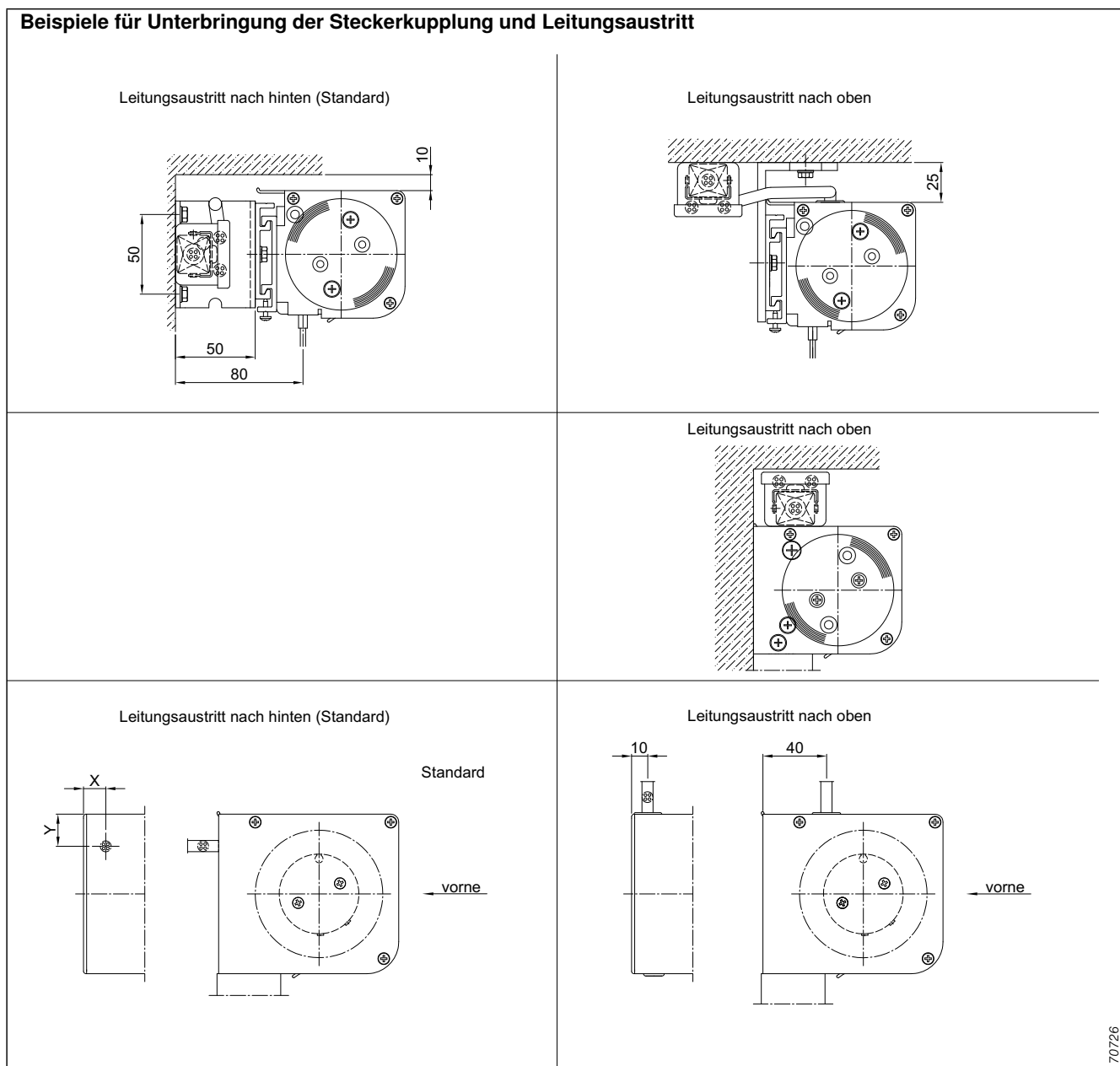
Abb. 125: Leitungsabgänge
