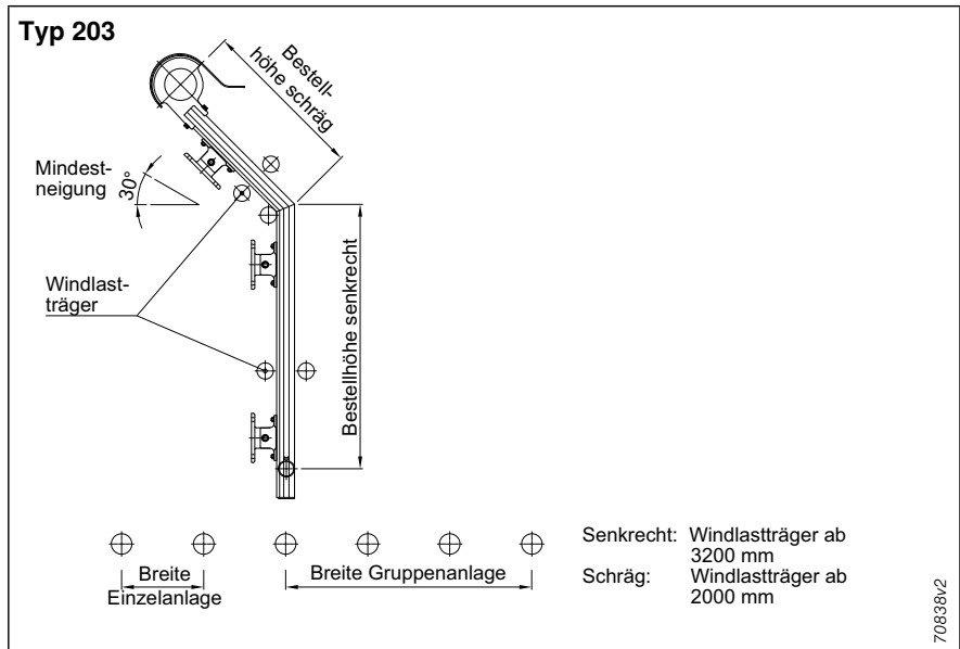
Abb. 168: Maßanleitung Fassaden-Markisen 203
