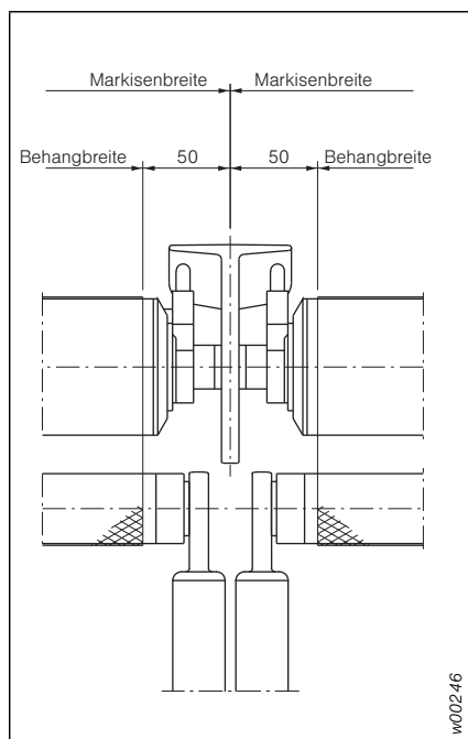
Abb. 146: Motor – Motor
