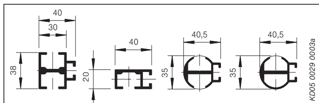
Abb. 255: Führungsprofile
