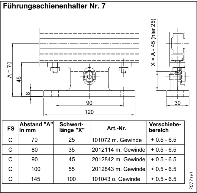
Abb. 271: Führungsschiene 40x20 mit Halter Nr. 7
