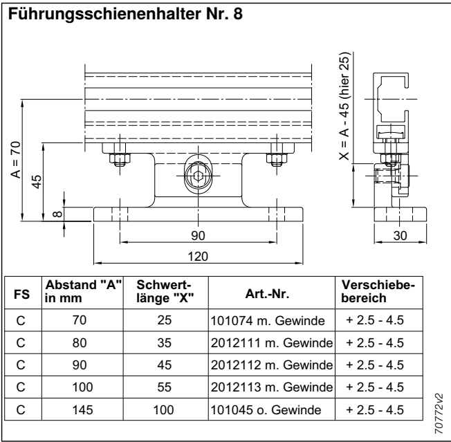
Abb. 272: Führungsschiene 40x20 mit Halter Nr. 8
