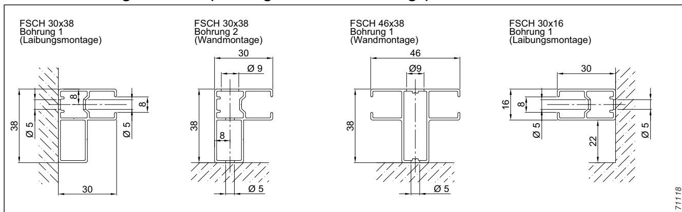
Abb. 111: Führungsschienenbohrungen
