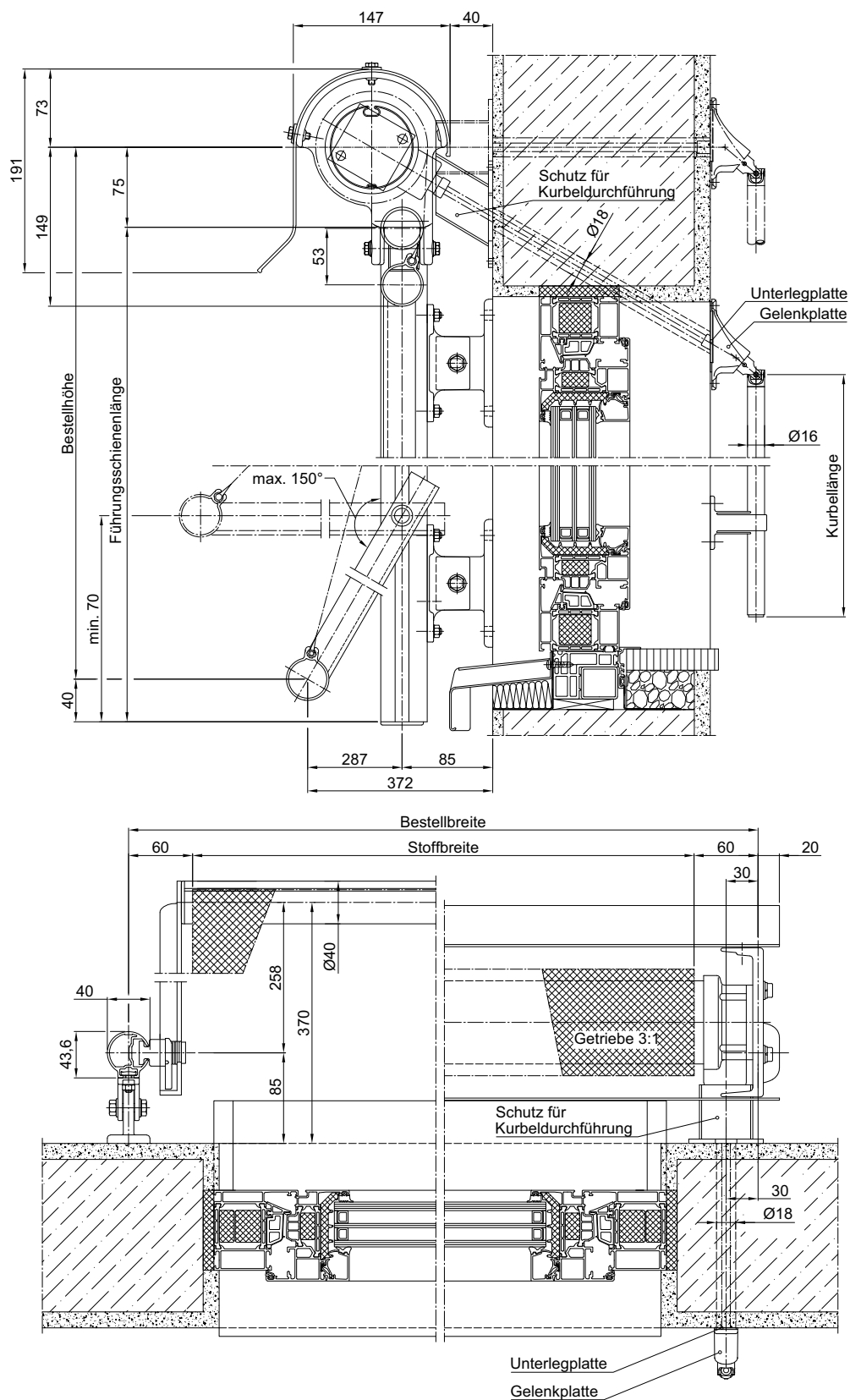
Abb. 245: Markisolette 101 mit Halbrundblende Typ 2.3
