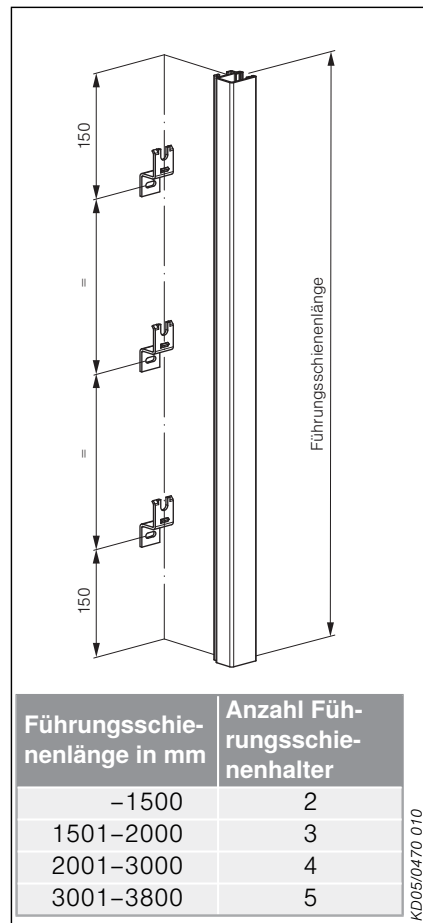
Abb. 67: Maßanleitung Führungsschie- nenhalter
