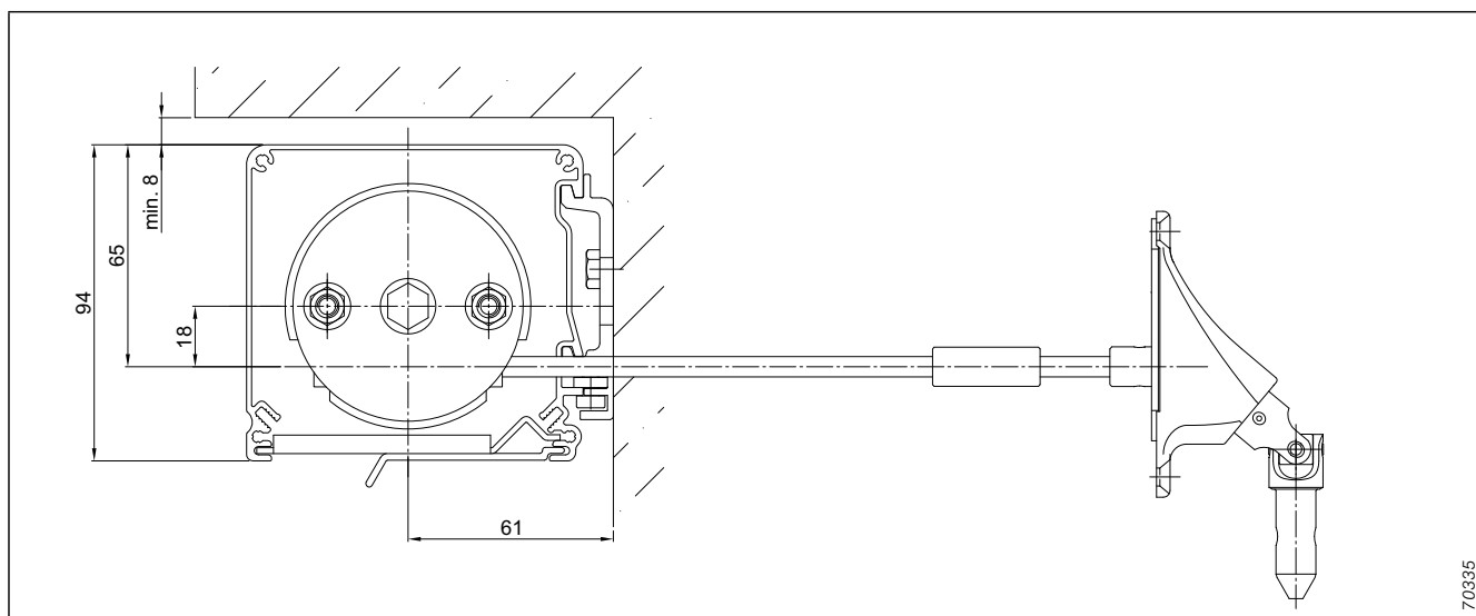
Abb. 38: Getriebeabgang 0°
