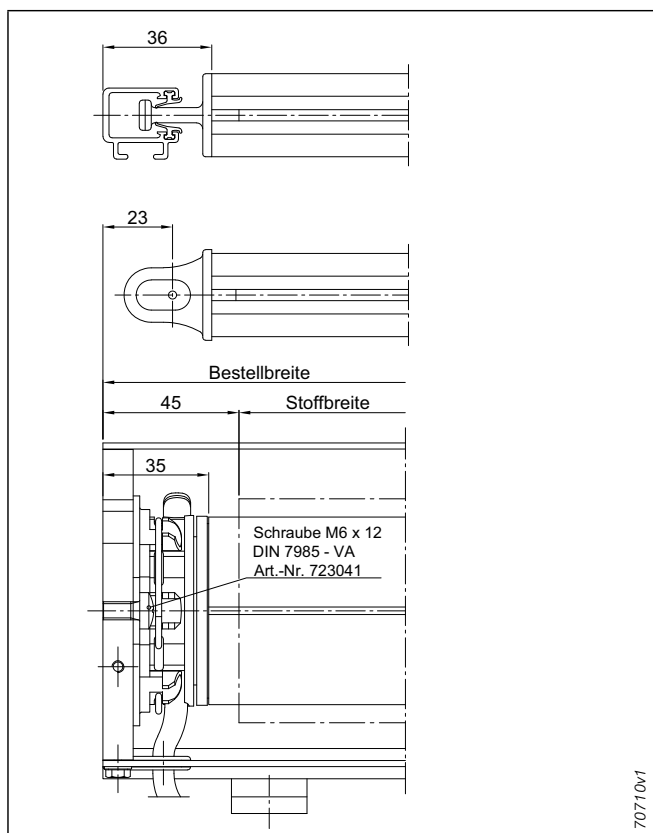
Abb. 75: Motorseite
