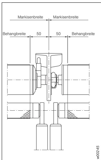
Abb. 145: Motor – Endlager
