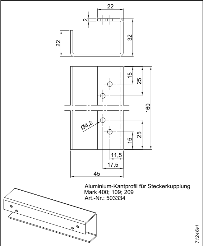
Abb. 287: Kantprofil für Steckerkuplung
