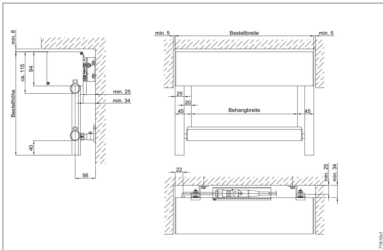
Abb. 42: Einzelanlage, Linksroller (auch als Rechtsroller lieferbar), Wandmontage, Führungsschiene, mit Leitungsaustritt hinten
