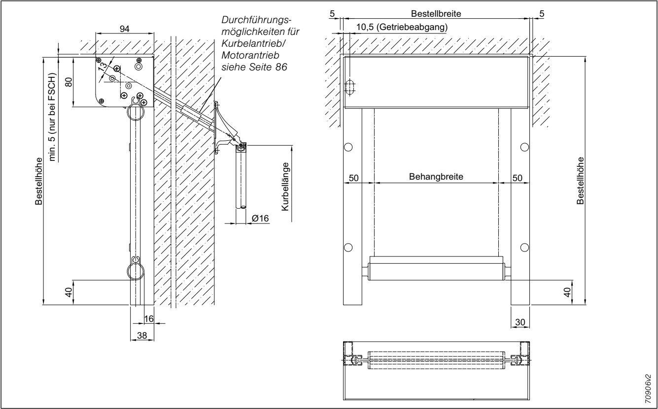
Abb. 115: Maßblatt
