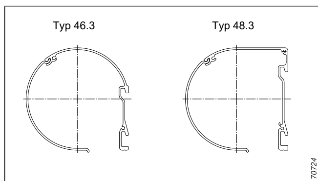
Abb. 63: Blenden
