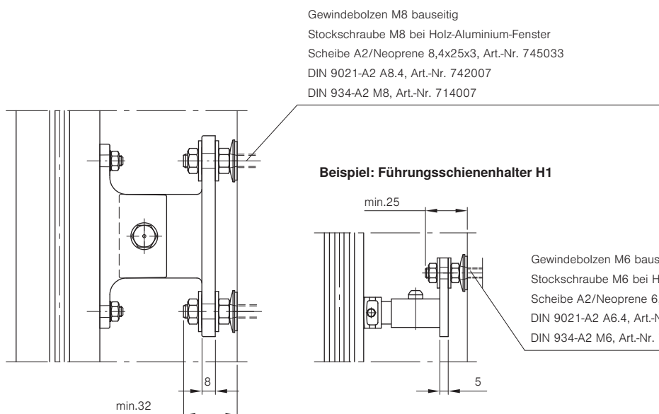
Abb. 278: WAREMA Befestigungssystem mit Anschlagmutter
