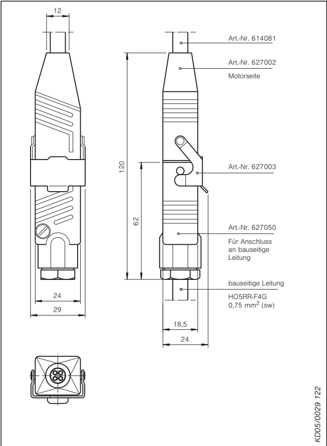
Abb. 285: Steckerkuplung
