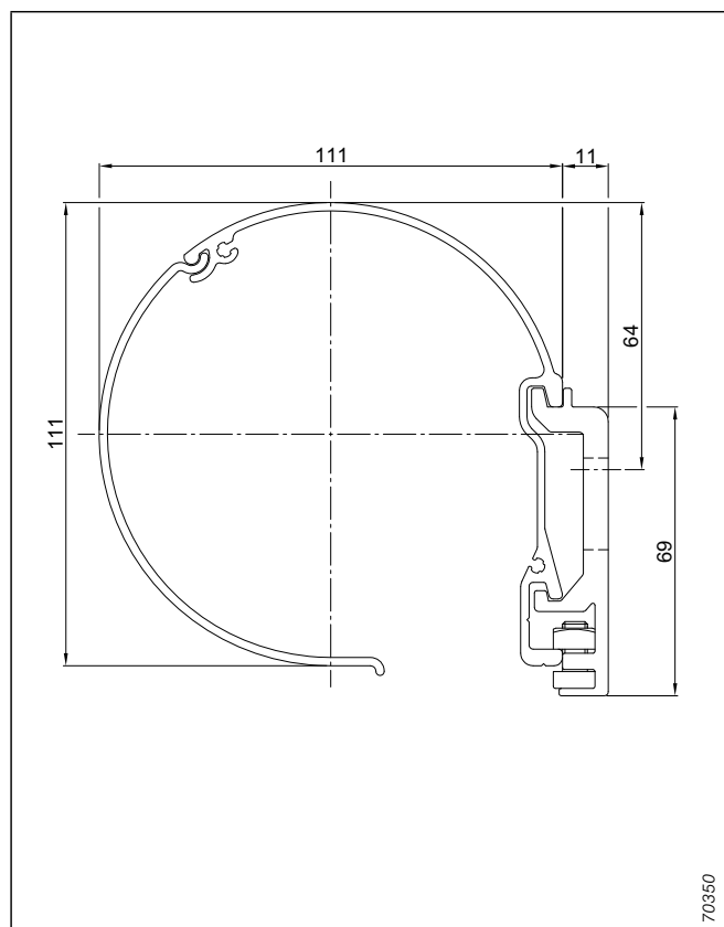
Abb. 83: Wandmontage Typ 46.3
