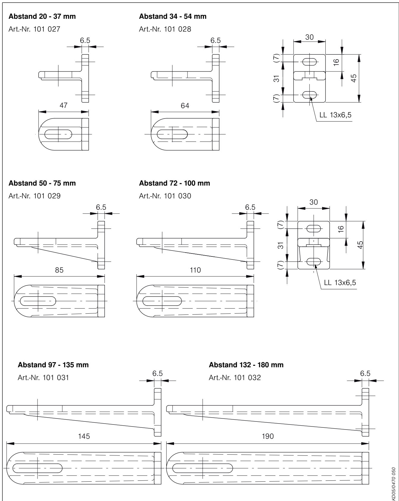
Abb. 96: Spannseilhalterübersicht
