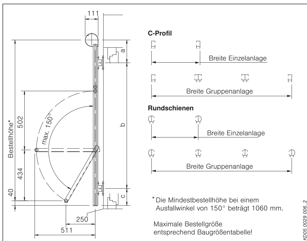
Abb. 257: Maßanleitung Markisolette 109
