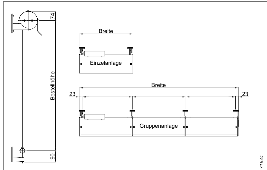
Abb. 208: Maßanleitung Fassaden-Markise 207
