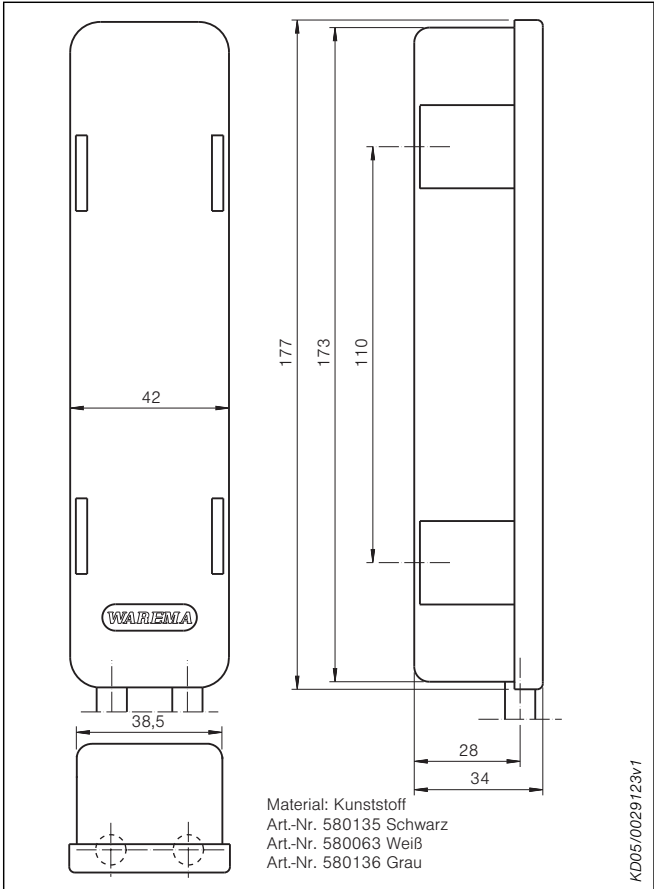
Abb. 286: Gehäuse für Steckerkuplung
