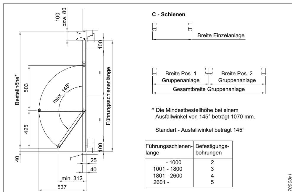
Abb. 269: Maßanleitung Markisolette 150
