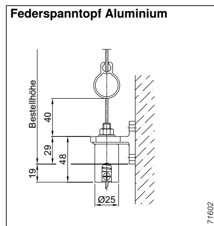
Abb. 8: Federspanntopf Aluminium
