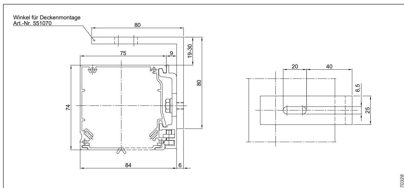
Abb. 25: Blende 470 – Deckenmontage
