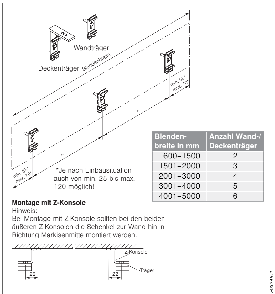
Abb. 4: Maßanleitung für Wand-/Deckenträger
