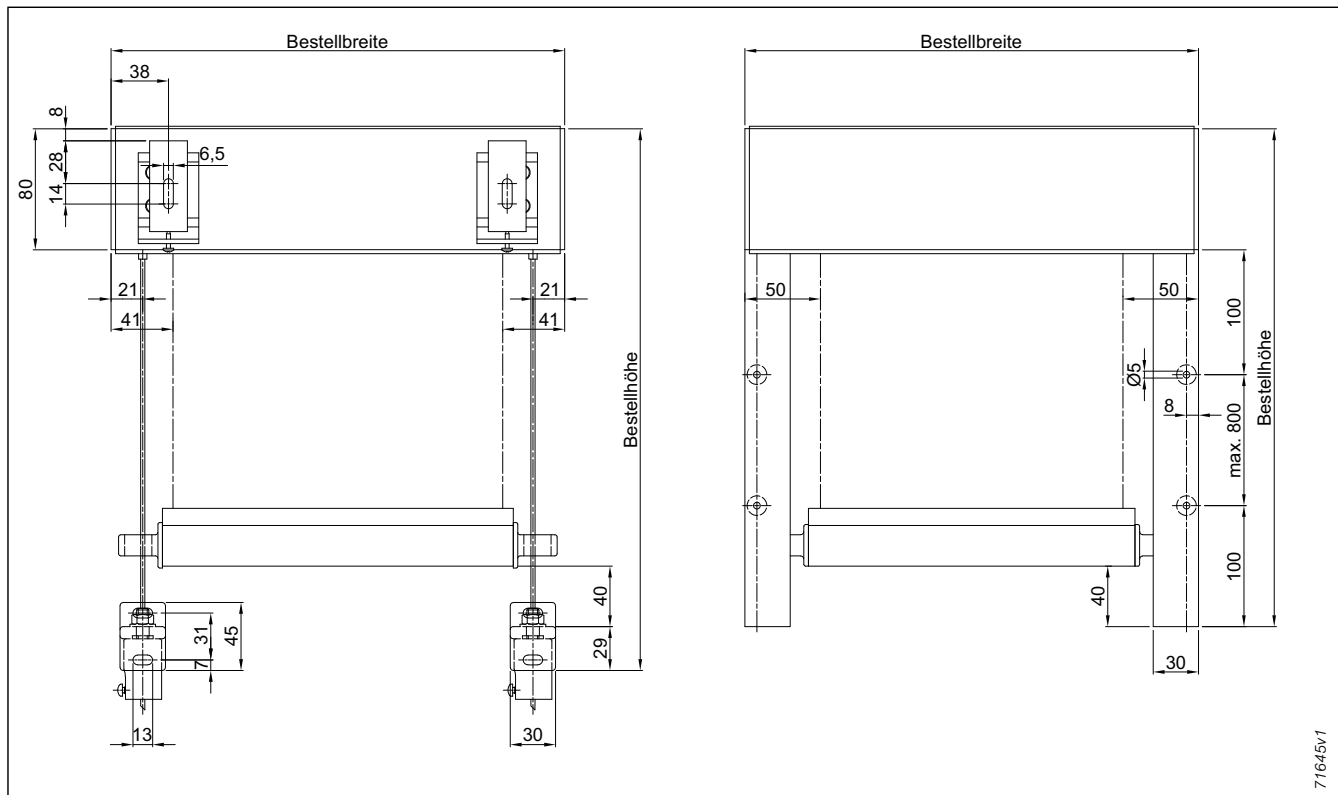
Abb. 113: Maßblatt
