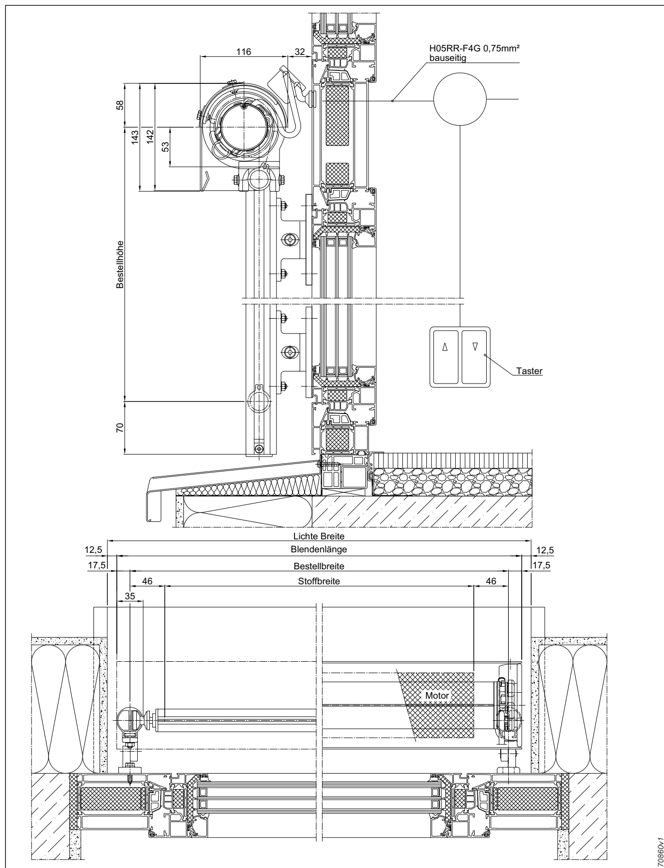
Abb. 229: Fassaden-Markise 209 mit Rundschiene Ø35 mm, Blende Typ 20.3
