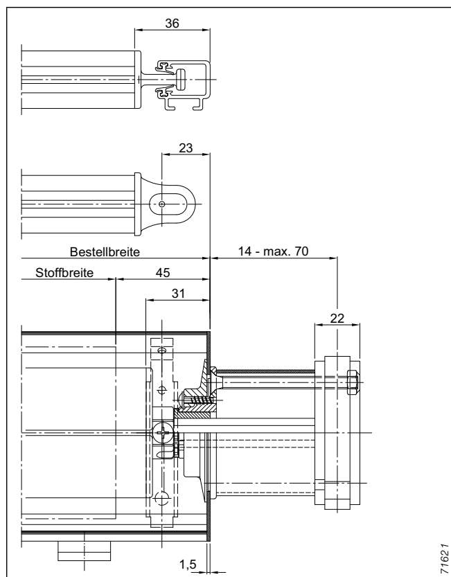
Abb. 58: Außenliegendes Getriebe
