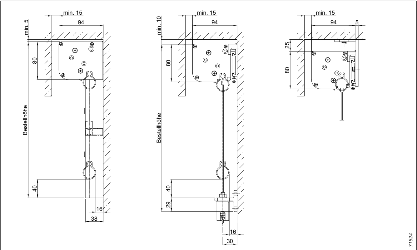
Abb. 116: Blende 80 – Montagesituation
