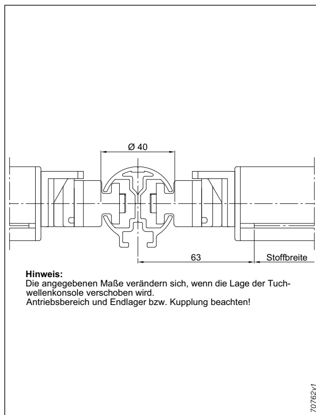
Abb. 251: Details Führungsschiene Ø40 mm – Stoffabzugsmaße für Typ 101
