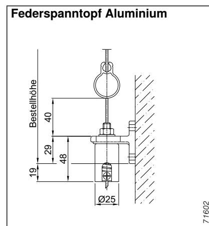
Abb. 33: Federspanntopf Aluminium
