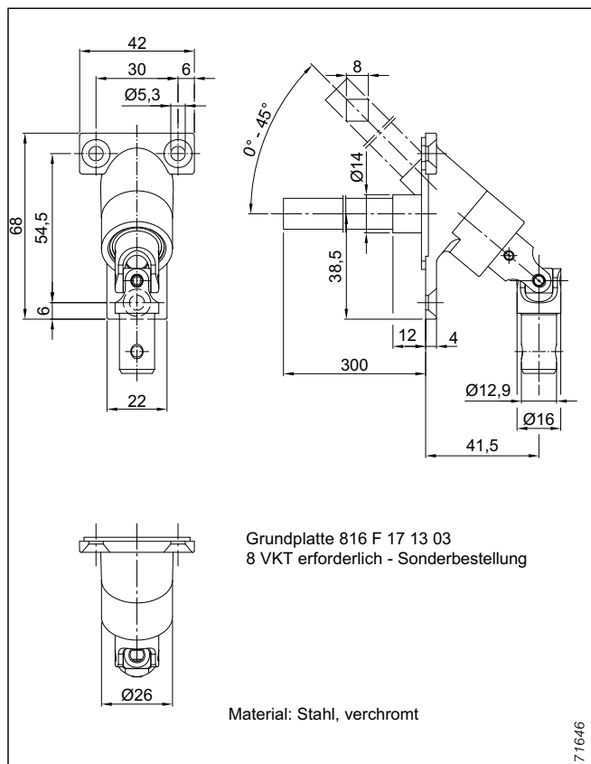
Abb. 192: Gelenkplatte 0°-45°
