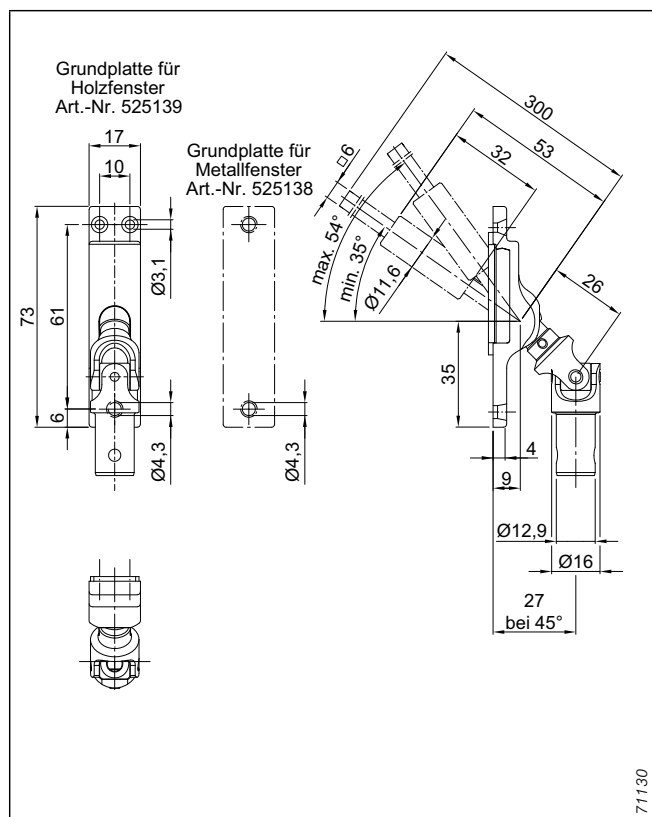
Abb. 102: Gelenkplatte 35°–54° für Kurbelantrieb mit thermischer Trennung
