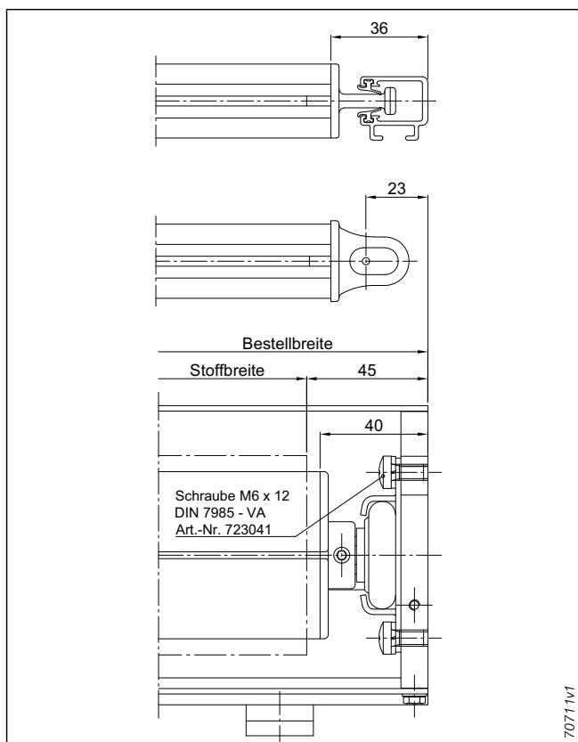
Abb. 76: Endlager
