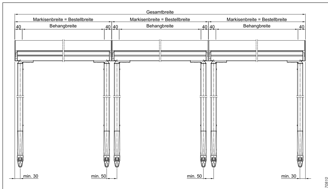
Abb. 130: Maßanleitung Fallarm-Markise 355 (gekuppelte Anlage)
