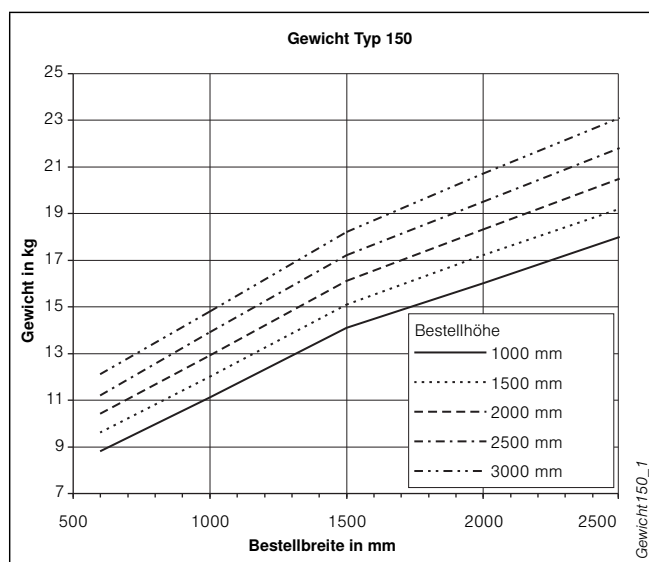
Abb. 268: Gewicht Typ 150
