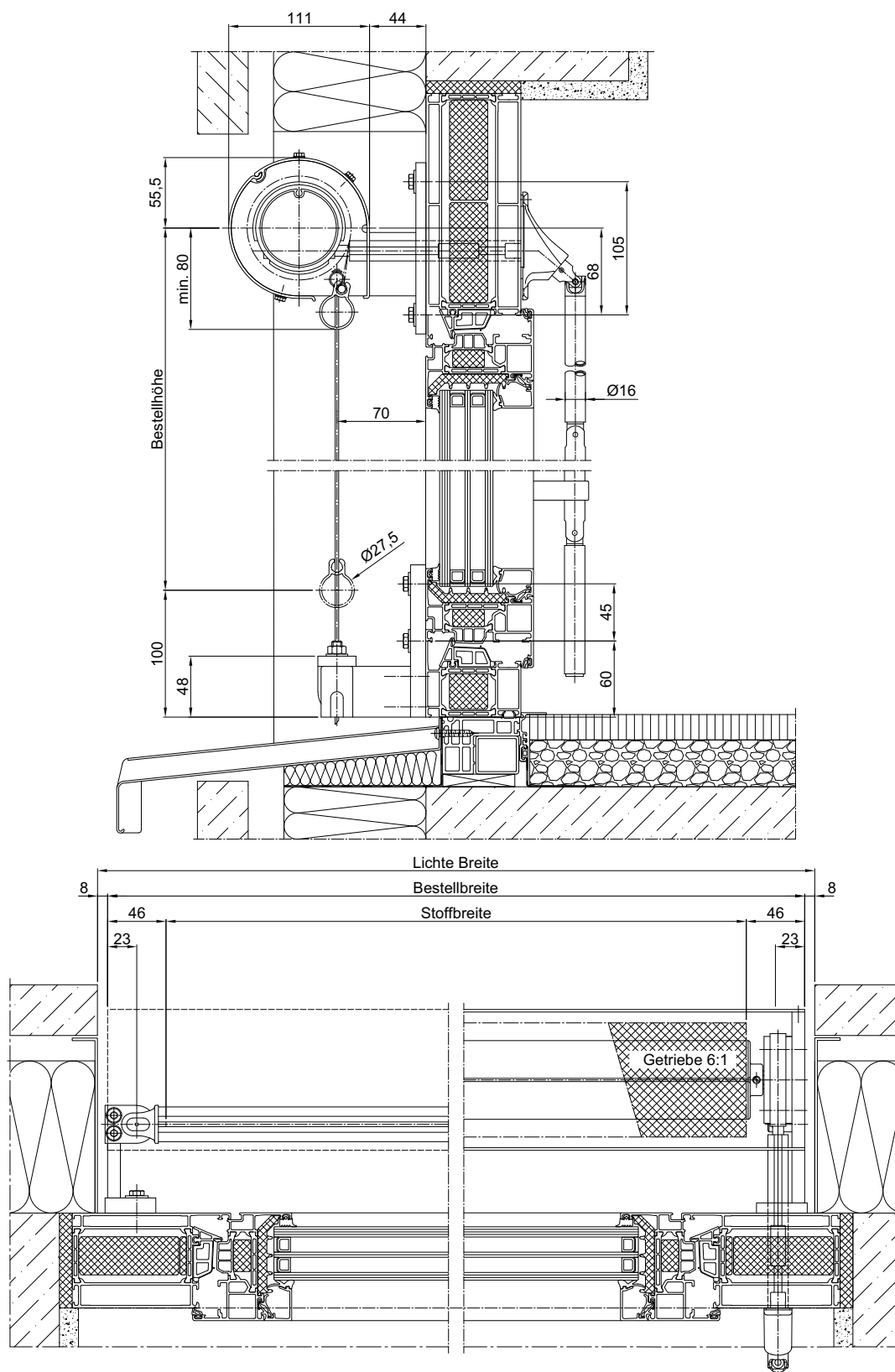
Abb. 232: Fassaden-Markise 209 mit Rundblende Typ 23.3 und Spannseil
