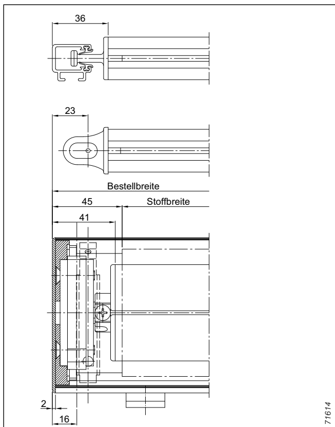
Abb. 51: Getriebe
