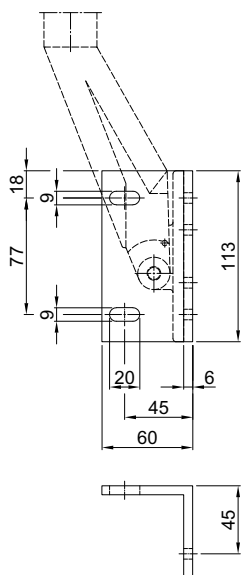
Abb. 152: Maßanleitung Fallarm-Markise 330 (Einzelanlage) – Wandmontage
