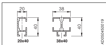
Abb. 267: Führungsschienen
