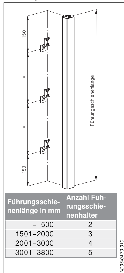
Abb. 5: Maßanleitung Führungsschienenhalter
