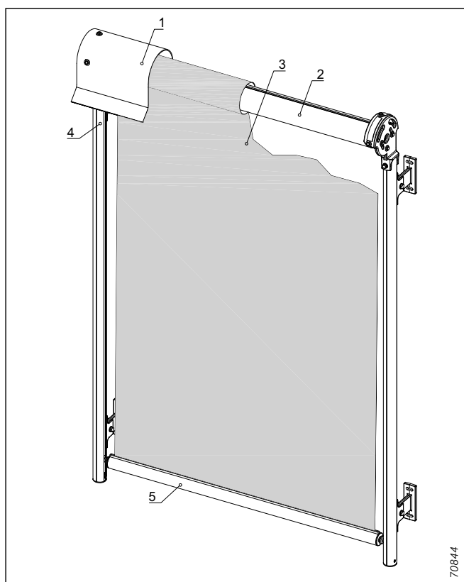
Abb. 163: Fassaden-Markise 201
