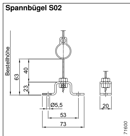
Abb. 68: Spannbügel S02
