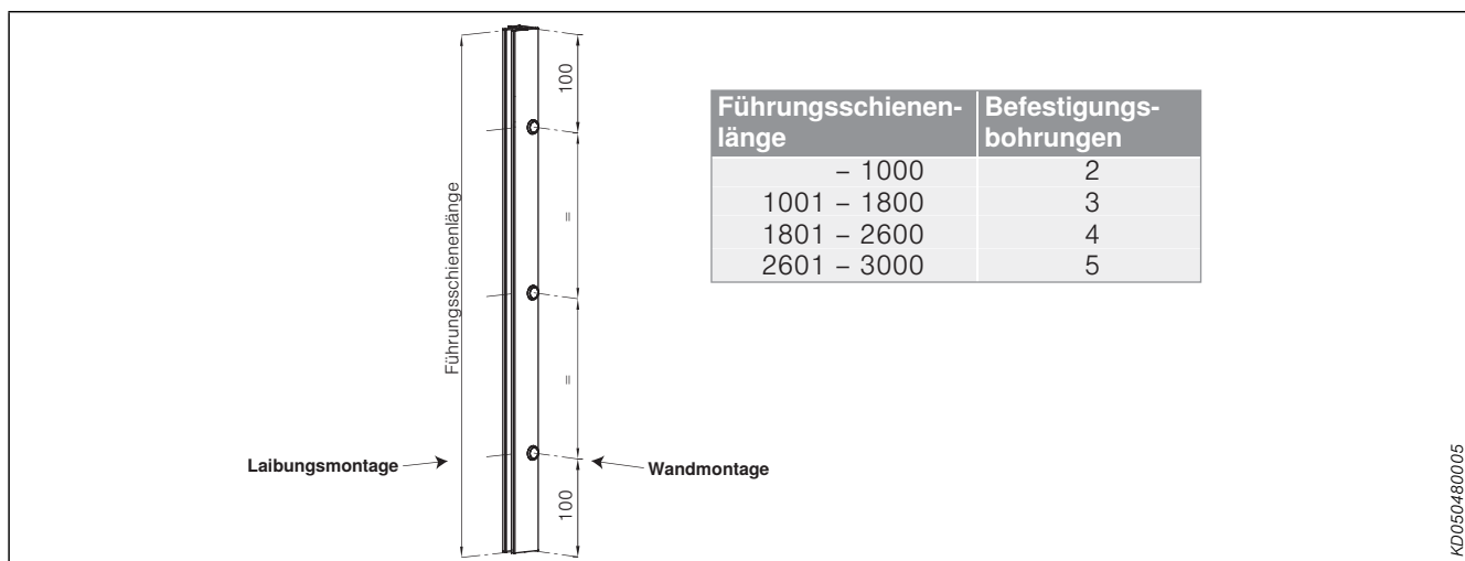
Abb. 110: Anzahl der Führungsschienenbohrungen
