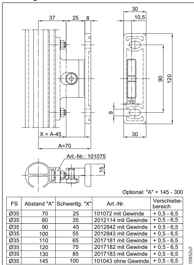
Abb. 200: Führungsschienenhalter Nr. 7
