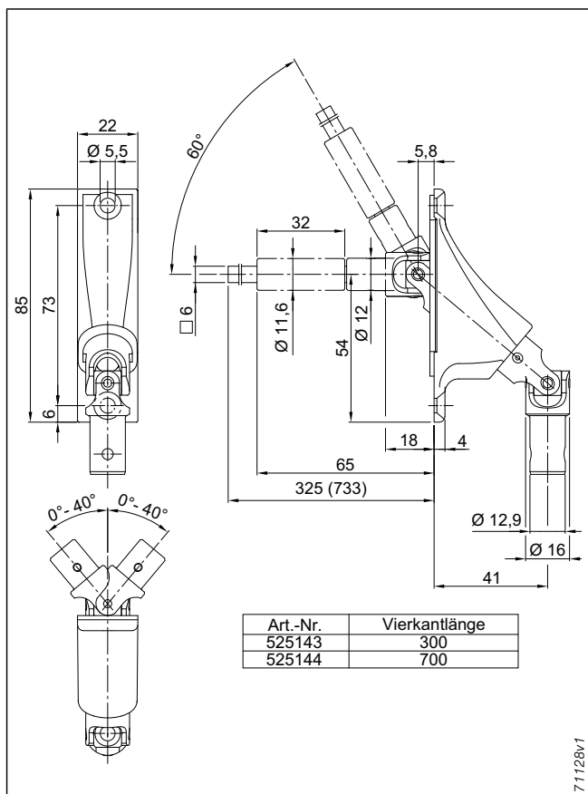
Abb. 236: Gelenkplatte 0°–60°
