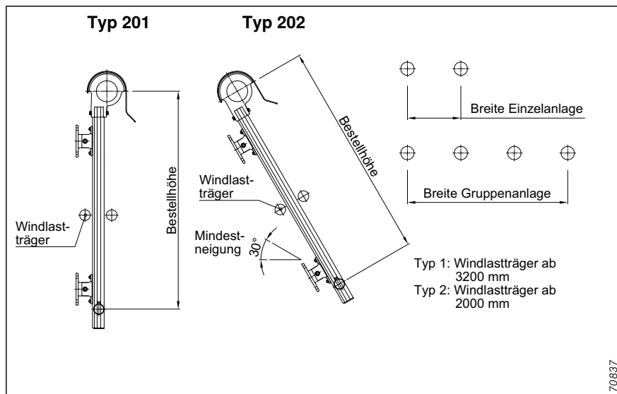
Abb. 167: Maßanleitung Fassaden-Markisen 201 und 202
