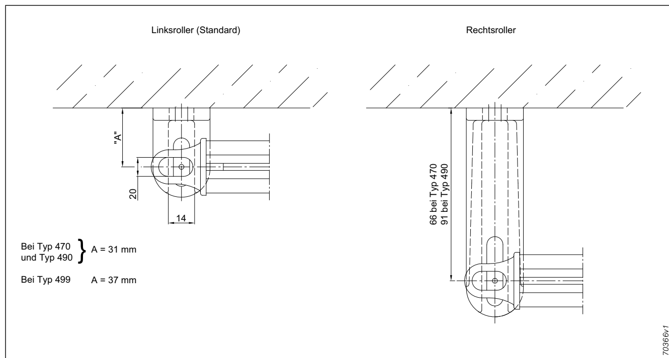
Abb. 93: Spannseilhalter
