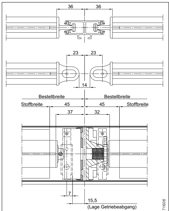
Abb. 20: Getriebe – Spindelsperre, durchgehende Blende, Standard
