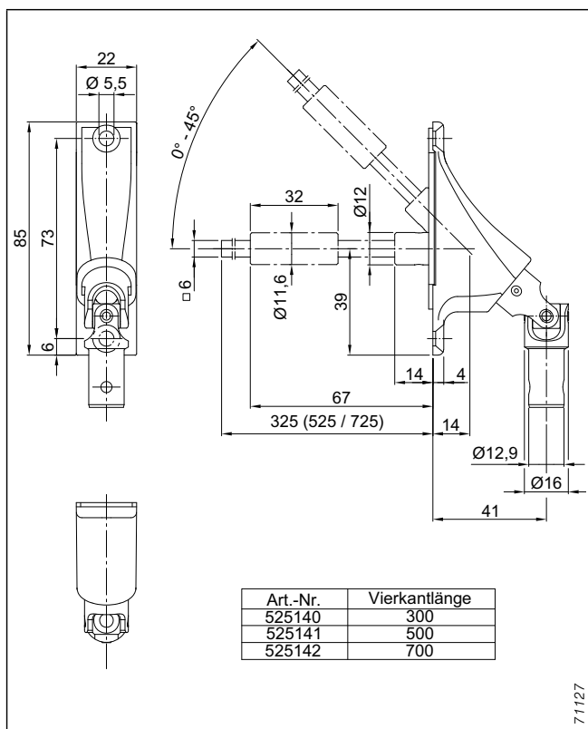
Abb. 234: Gelenkplatte 0°–45°
