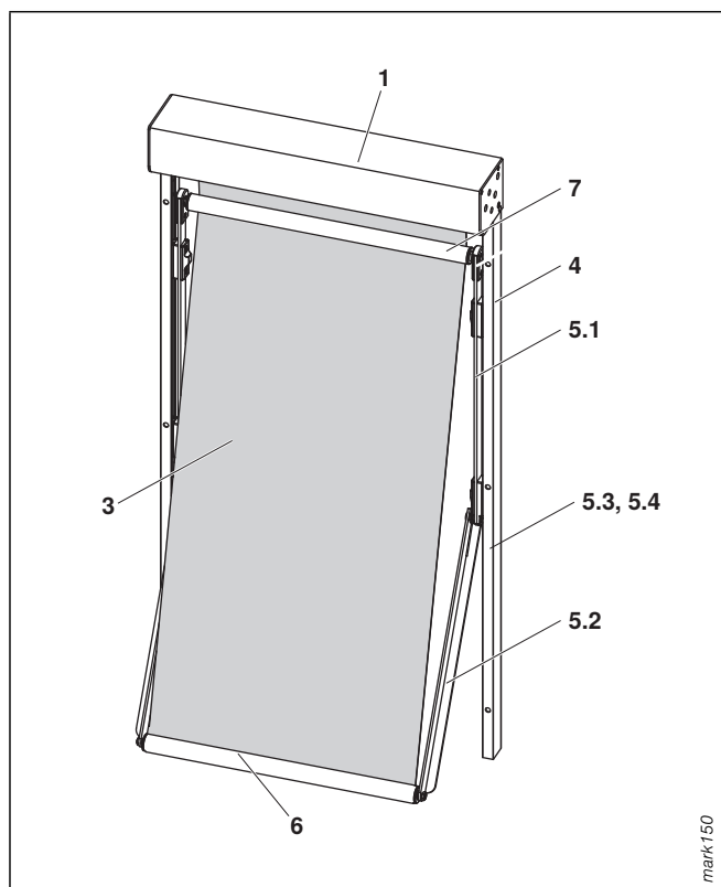
Abb. 265: Markisolette 150
