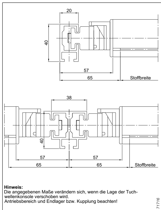
Abb. 250: Details Führungsschienen 20/40 und 38/40 – Stoffabzugsmaße für Typ 101
