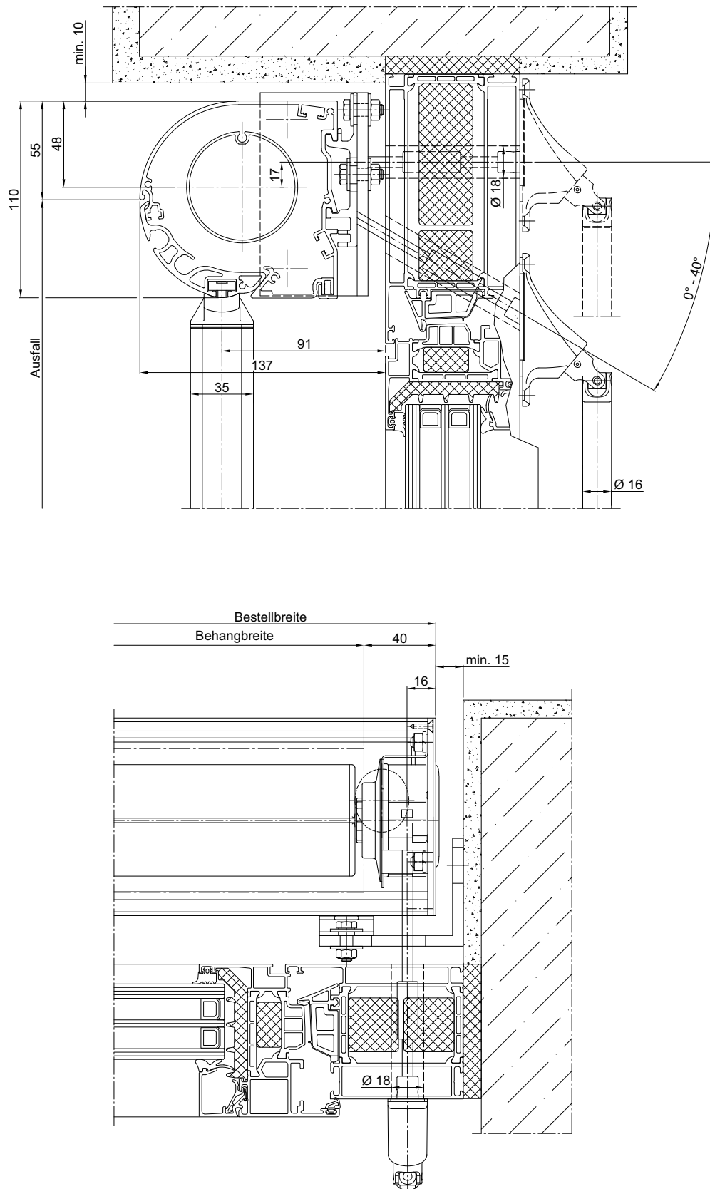
Abb. 135: Fallarm-Markise 355: Kurbelbedienung von innen bei Befestigung in der Laibung
