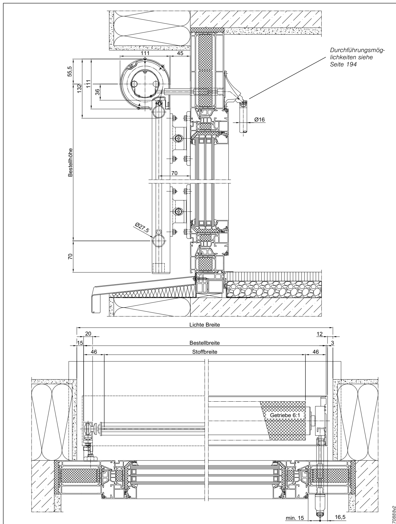
Abb. 225: Fassaden-Markise 209 mit Führungsschiene 20x40 mm, Getriebe 6:1, Blende Typ 23.3
