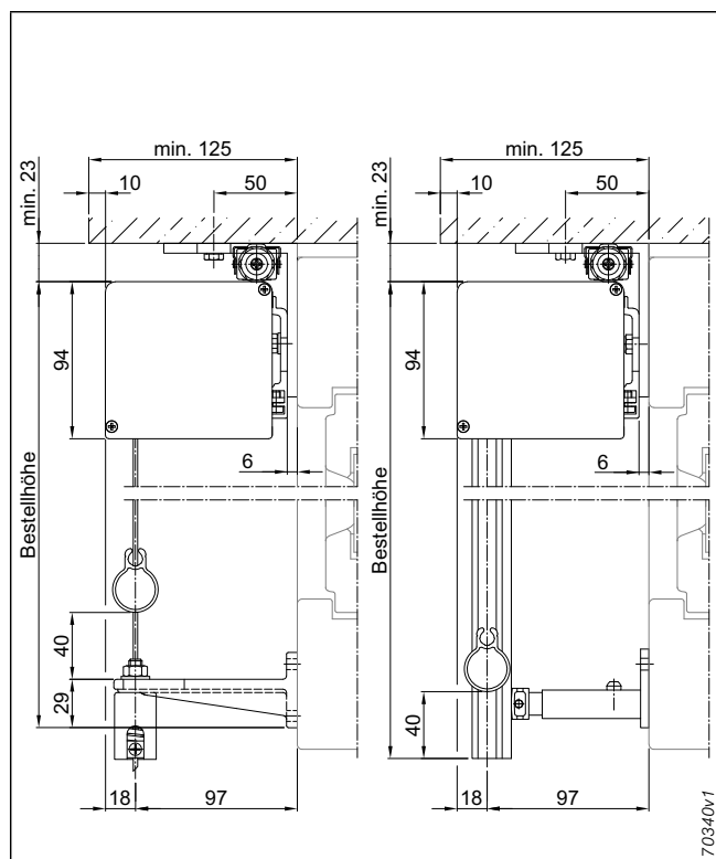
Abb. 44: Rechtsroller (auch als Linksroller lieferbar), Deckenmontage, Seilführung, Führungsschiene
