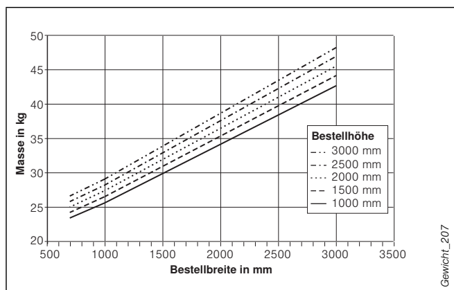
Abb. 207: Gewichte
