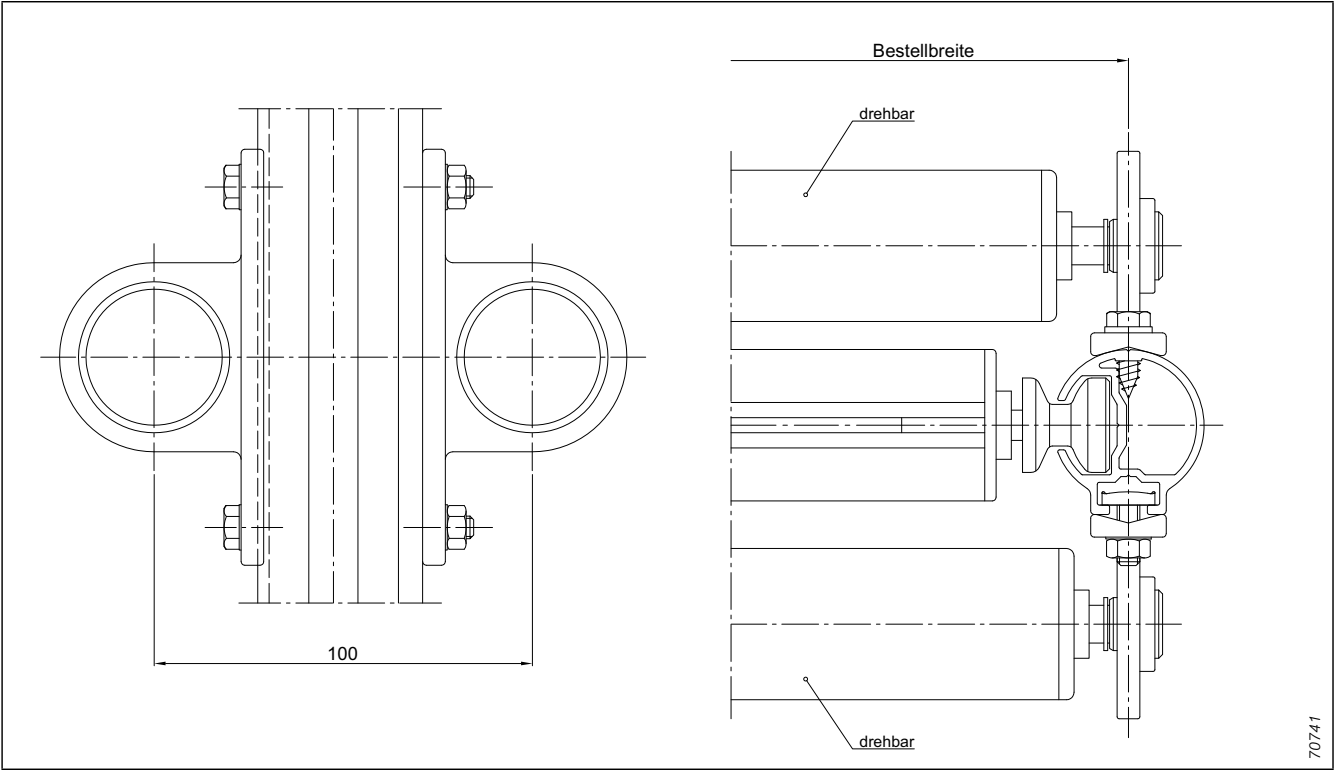
Abb. 189: Windlastträger
