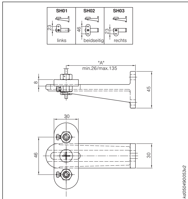
Abb. 97: Spannseilhalter SH01, SH02 und SH03 mit Querplatte
