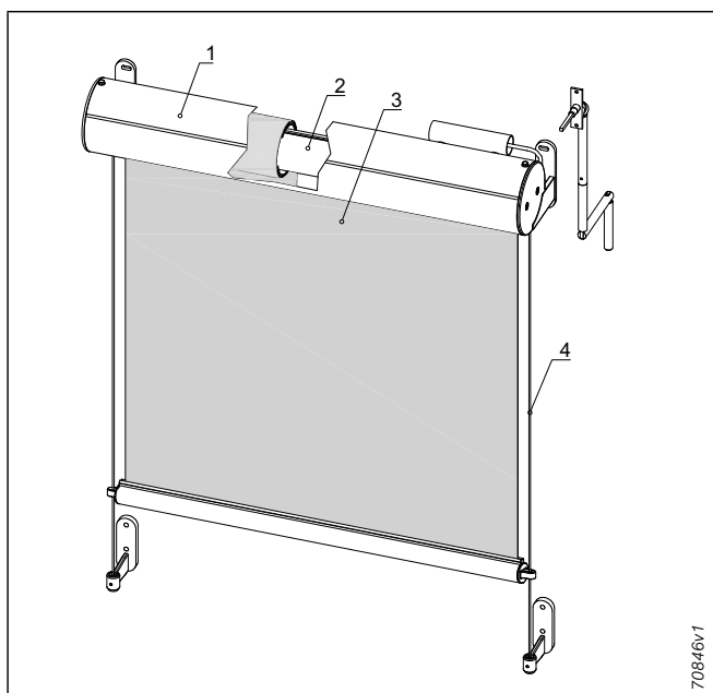
Abb. 204: Fassaden-Markise 207
