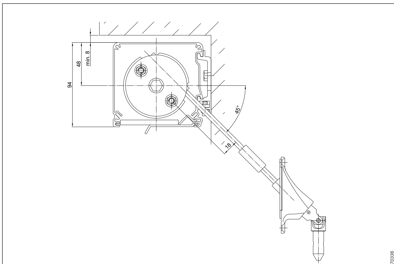
Abb. 39: Getriebeabgang 1-45°
