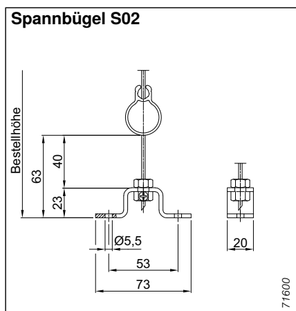
Abb. 6: Spannbügel S02
