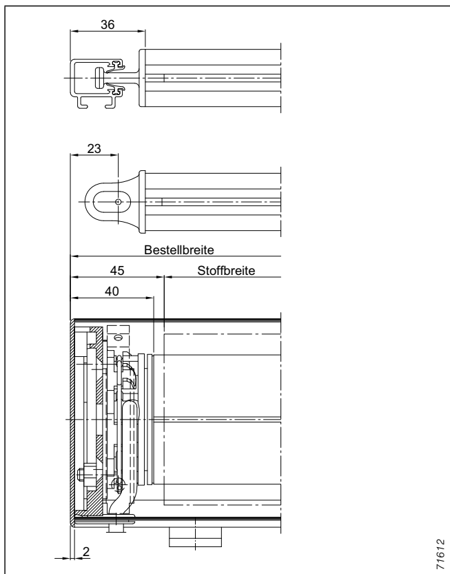
Abb. 49: Motorseite
