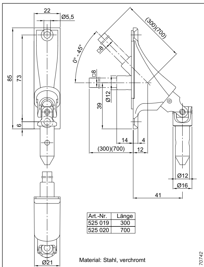
Abb. 191: Gelenkplatte 0°-45°
