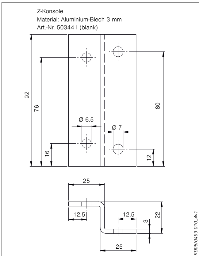
Abb. 88: Z-Konsole für Distanz-Montage bei Wandträger
