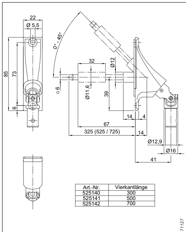
Abb. 103: Gelenkplatte 0°–45° für Kurbelantrieb mit thermischer Trennung
