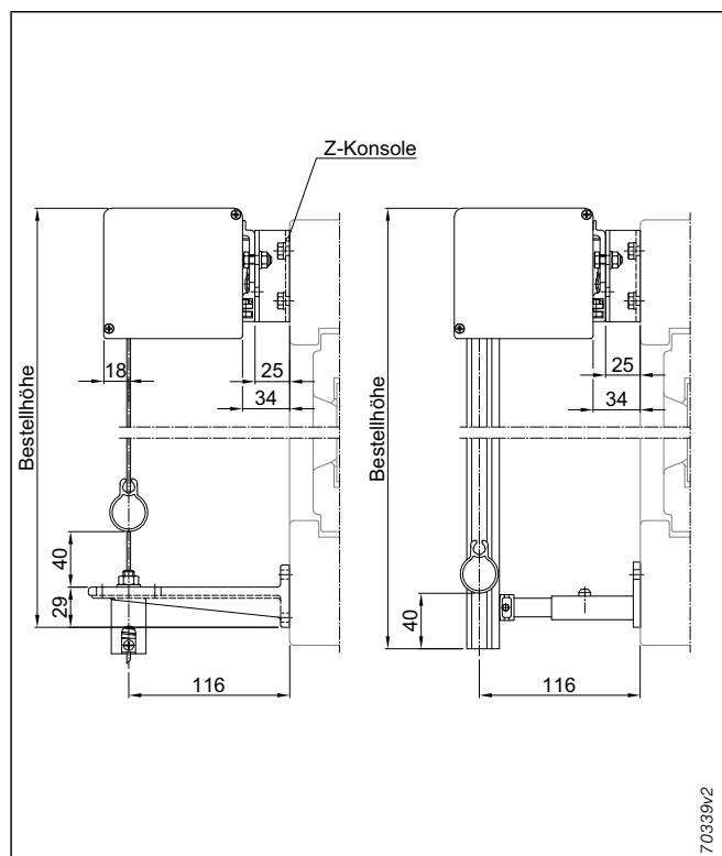
Abb. 43: Rechtsroller (auch als Linksroller lieferbar), Wandmontage, Seilführung, Führungsschiene
