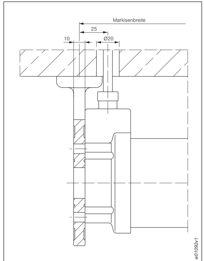
Abb. 142: Kurbeldurchführung
