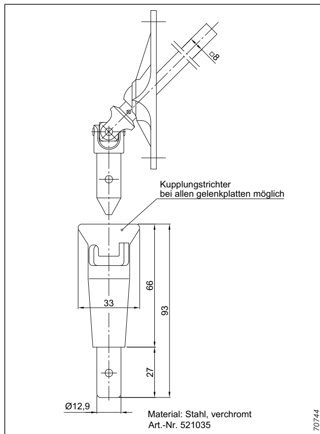
Abb. 195: Kupplungstrichter
