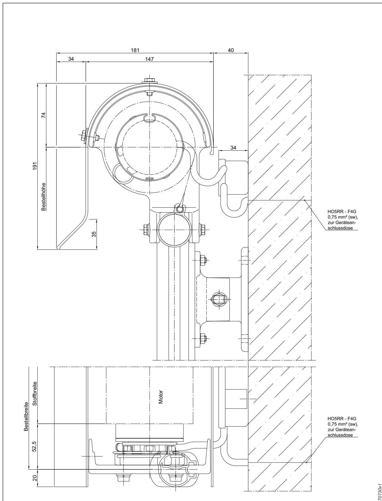
Abb. 177: Fassade-Markise 201 mit Halbrundblende Typ 2.3
