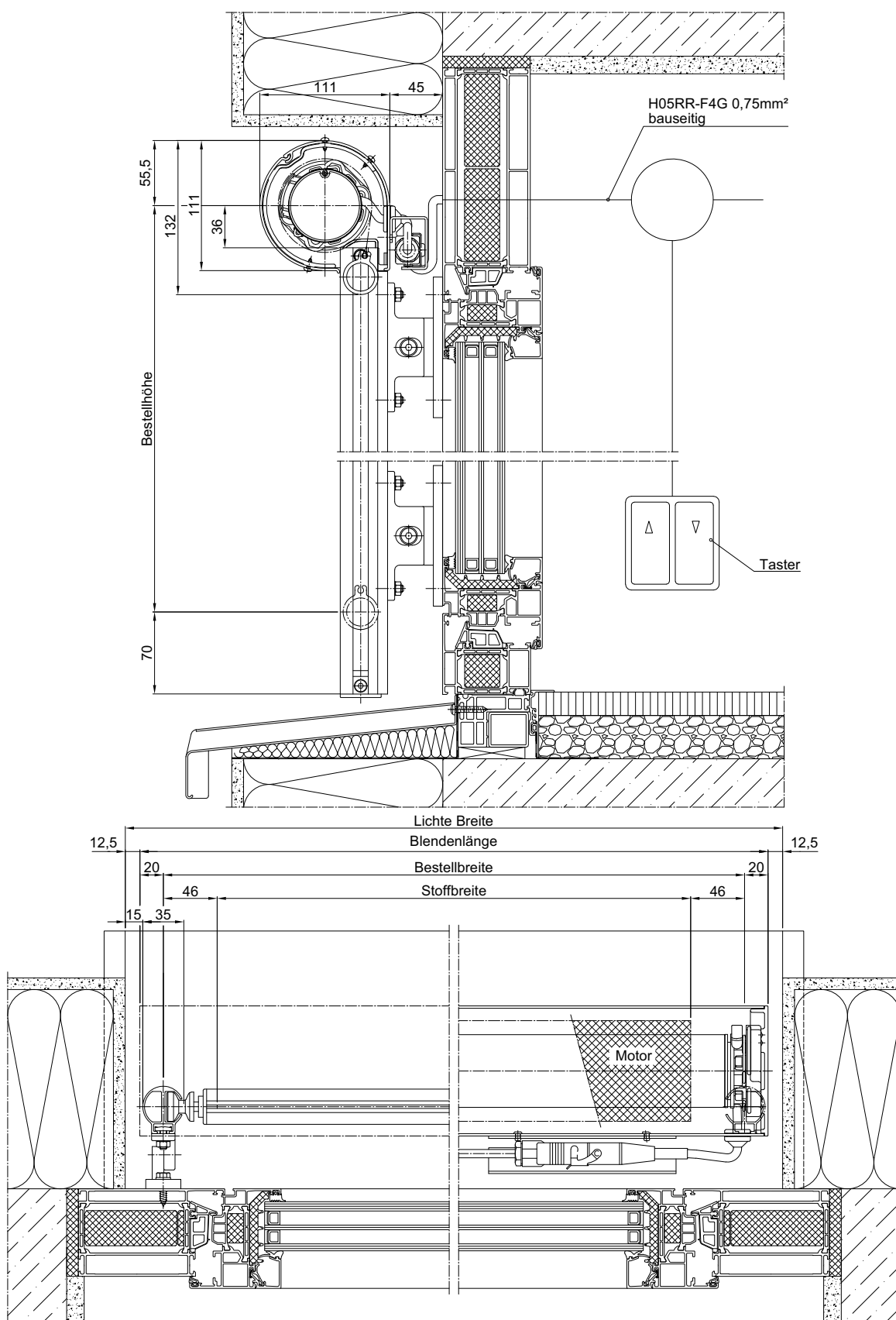
Abb. 228: Fassaden-Markise 209 mit Rundschiene Ø35 mm, Blende Typ 23.3
