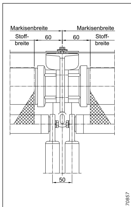
Abb. 149: Getriebe – Getriebe
