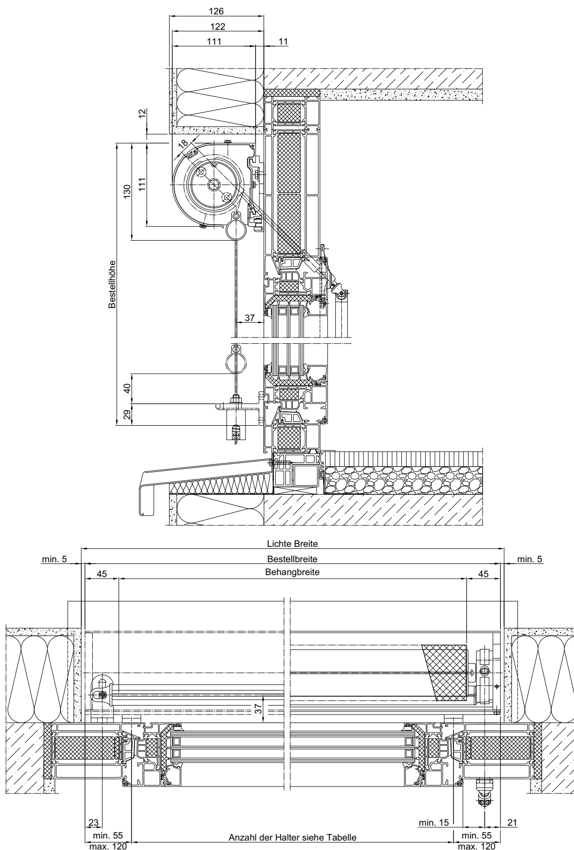
Abb. 71: Senkrecht-Markise 499 – Seilführung, Kurbelantrieb
