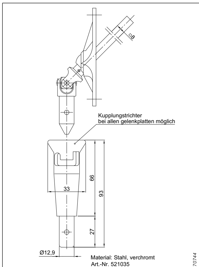
Abb. 238: Kuplungstrichter
