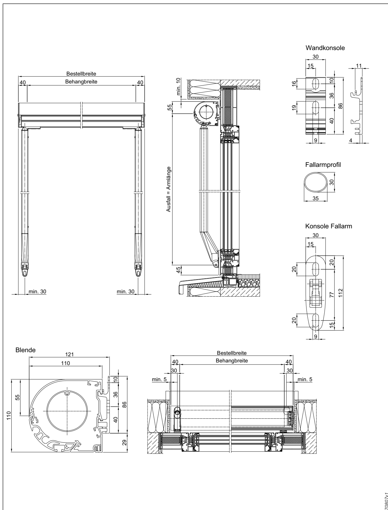
Abb. 129: Maßanleitung Fallarm-Markise 355 (Einzelanlage) – Wandmontage
