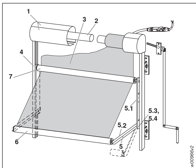
Abb. 253: Markisolette 109
