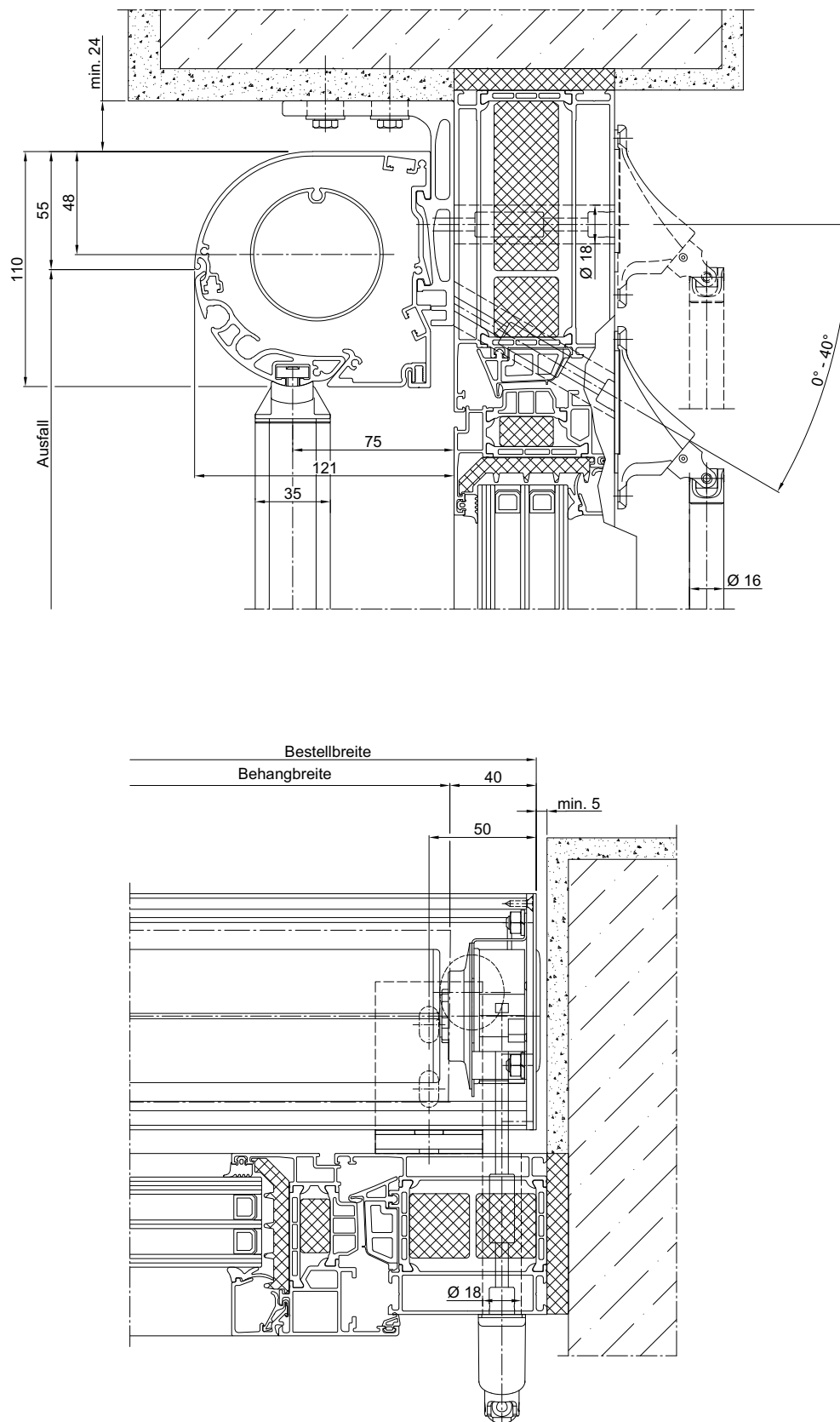
Abb. 134: Fallarm-Markise 355: Kurbelbedienung von innen bei Befestigung an der Decke
