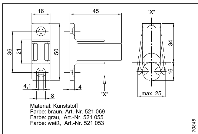
Abb. 196: Kurbelhalter
