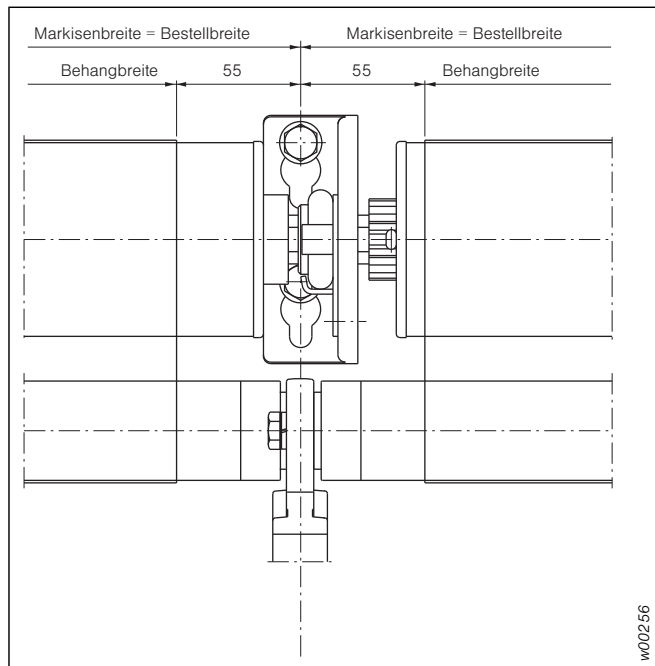
Abb. 157: Maanleitung
