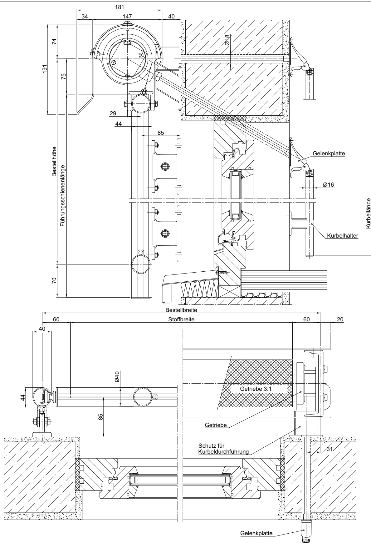
Abb. 171: Fassaden-Markise 201 mit Halbrundblende Typ 2.3; Kurbelantrieb
