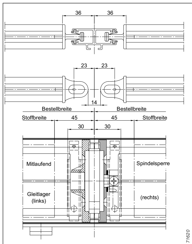
Abb. 57: Mittenge triebe
