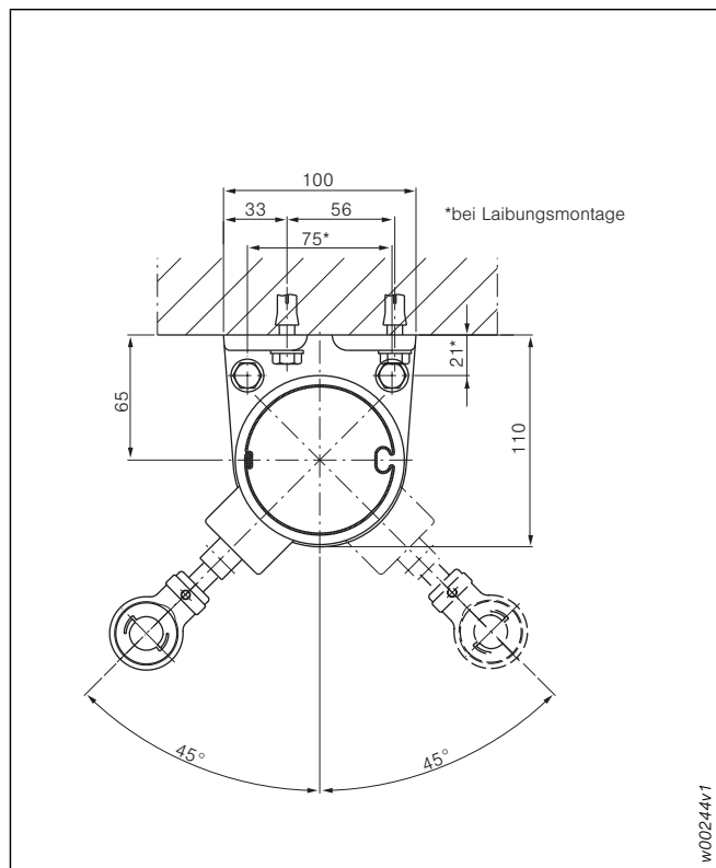
Abb. 154: Decken- und Laibungsmontage mit außenliegendem Kurbelantrieb
