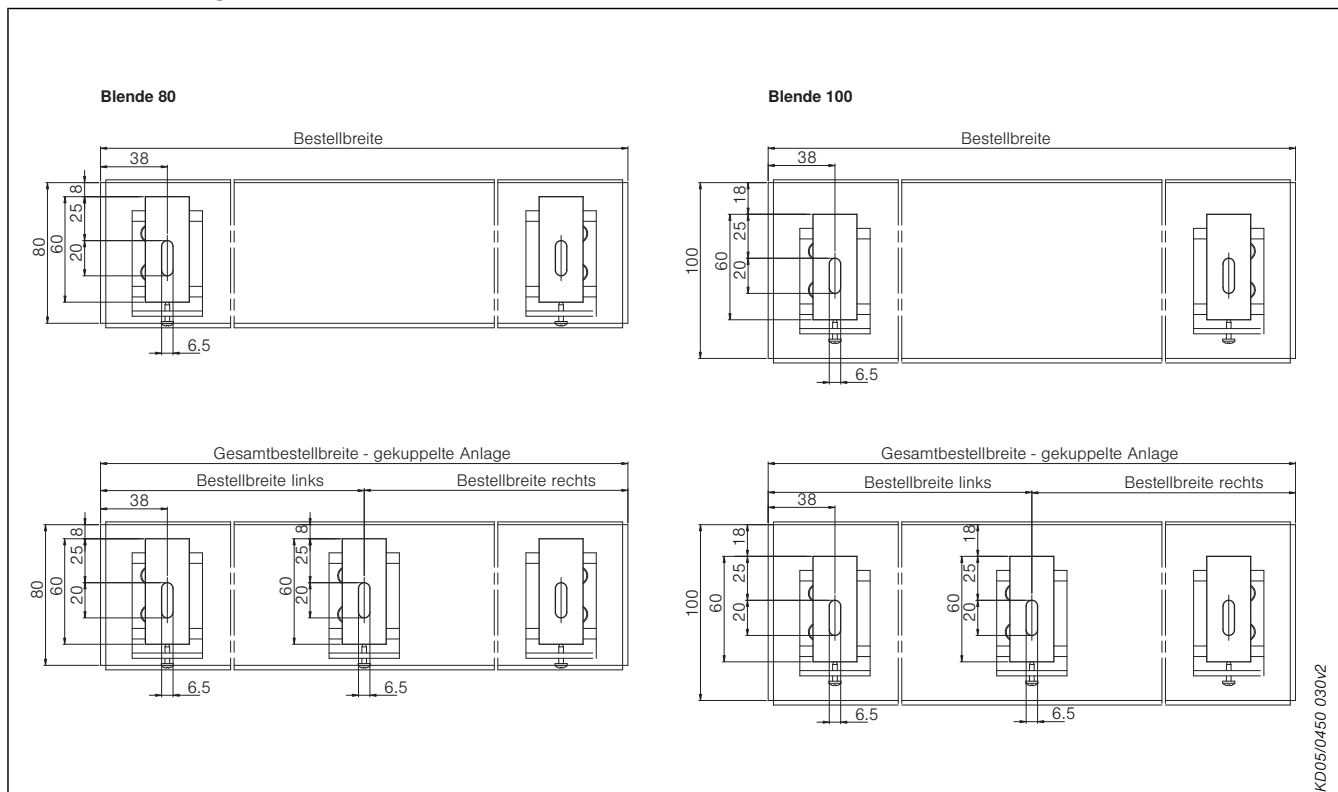
Abb. 114: Blendenmontage
