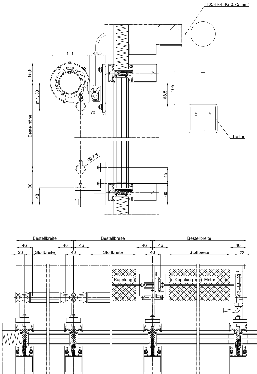
Abb. 230: Fassaden-Markise 209 mit Rundblende Typ 23.3 und Spannseil
