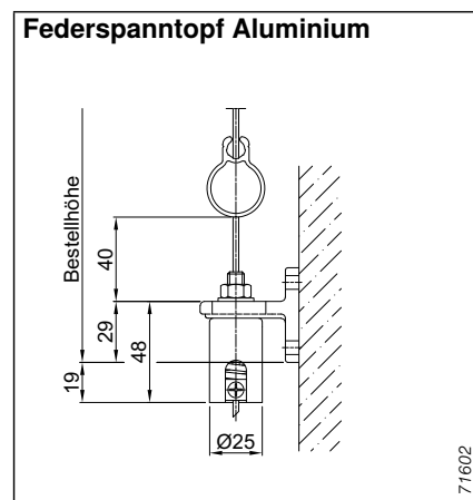
Abb. 70: Federspanntopf Aluminium
