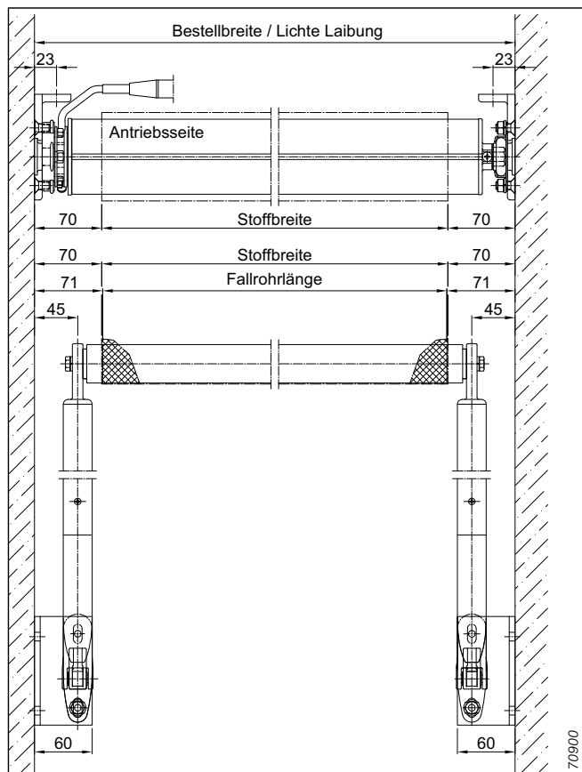
Abb. 156: Maßangaben
