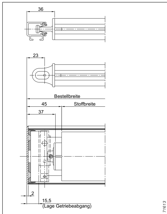
Abb. 50: Endlager
