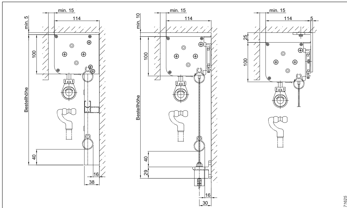
Abb. 117: Blende 100 – Montagesituation
