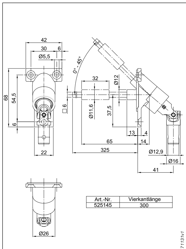
Abb. 235: Gelenkplatte 0°–45°
