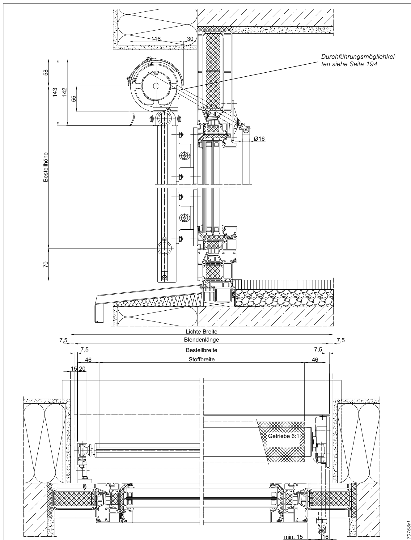
Abb. 226: Fassaden-Markise 209 mit Führungsschiene 20x40 mm, Blende Typ 20.3
