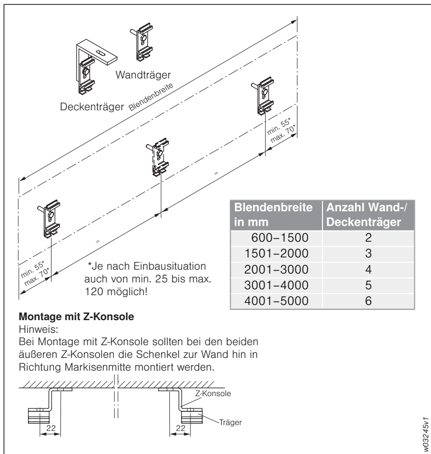
Abb. 29: Maßanleitung für Wand-/Deckenträger
