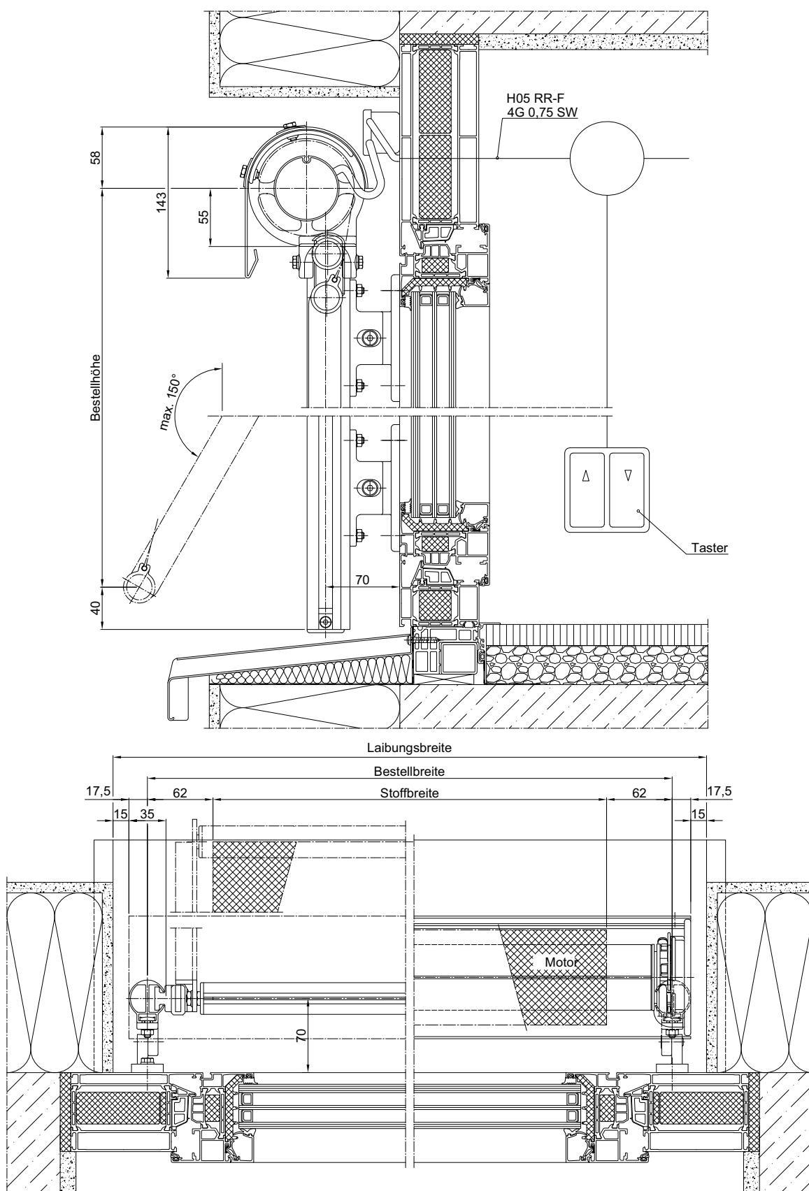
Abb. 261: Markisolette 109 mit Rundführungsschiene Ø35 mm, Blende Typ 20.3
