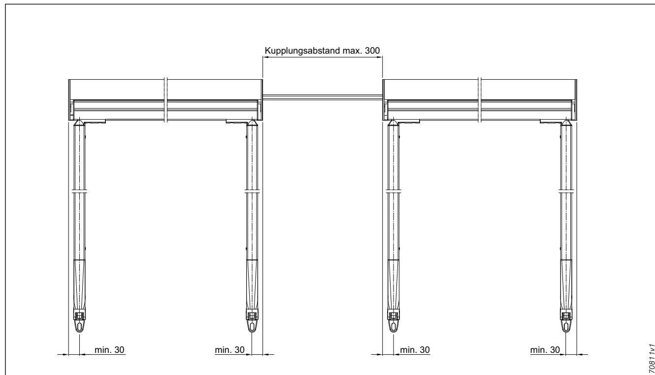
Abb. 131: Kupplungsabstand Fallarm-Markise 355
