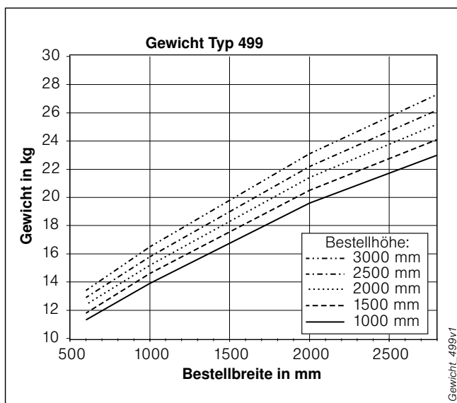
Abb. 64: Gewicht 499
