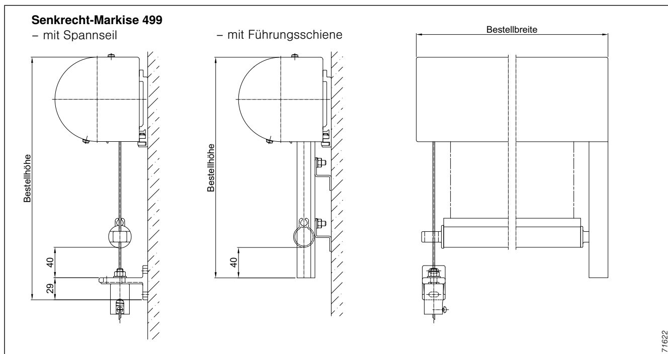
Abb. 65: Maßanleitung Senkrecht-Markise 499
