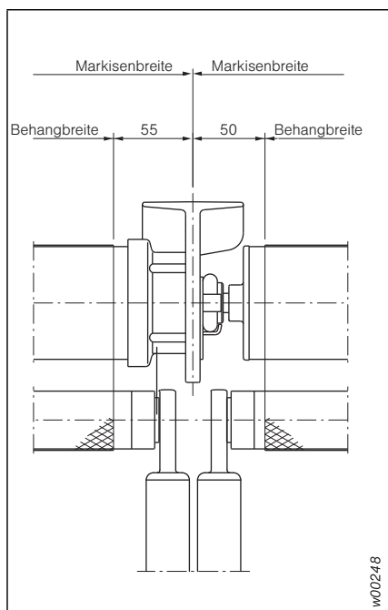
Abb. 148: Getriebe – Endlager
