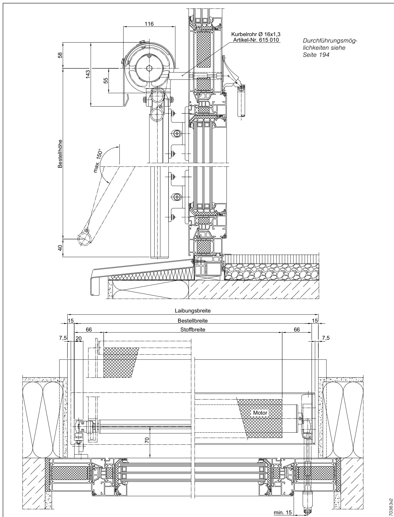
Abb. 259: Markisolette 109 mit Führungsschiene 20x40 mm, Blende Typ 20.3
