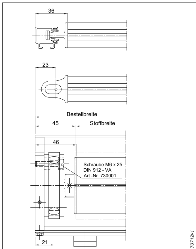
Abb. 77: Getriebe
