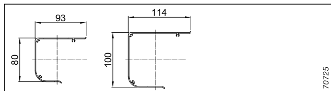
Abb. 106: Blenden
