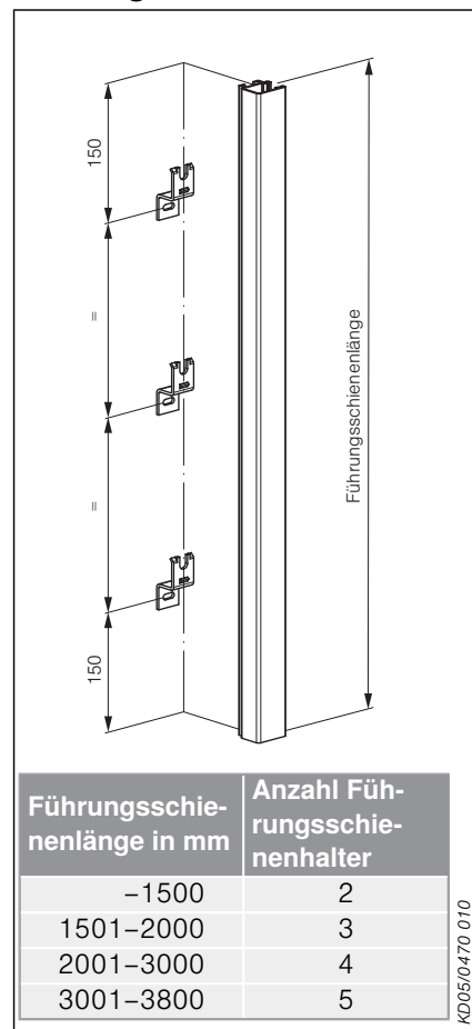
Abb. 30: Maßanleitung Führungsschienenhalter
