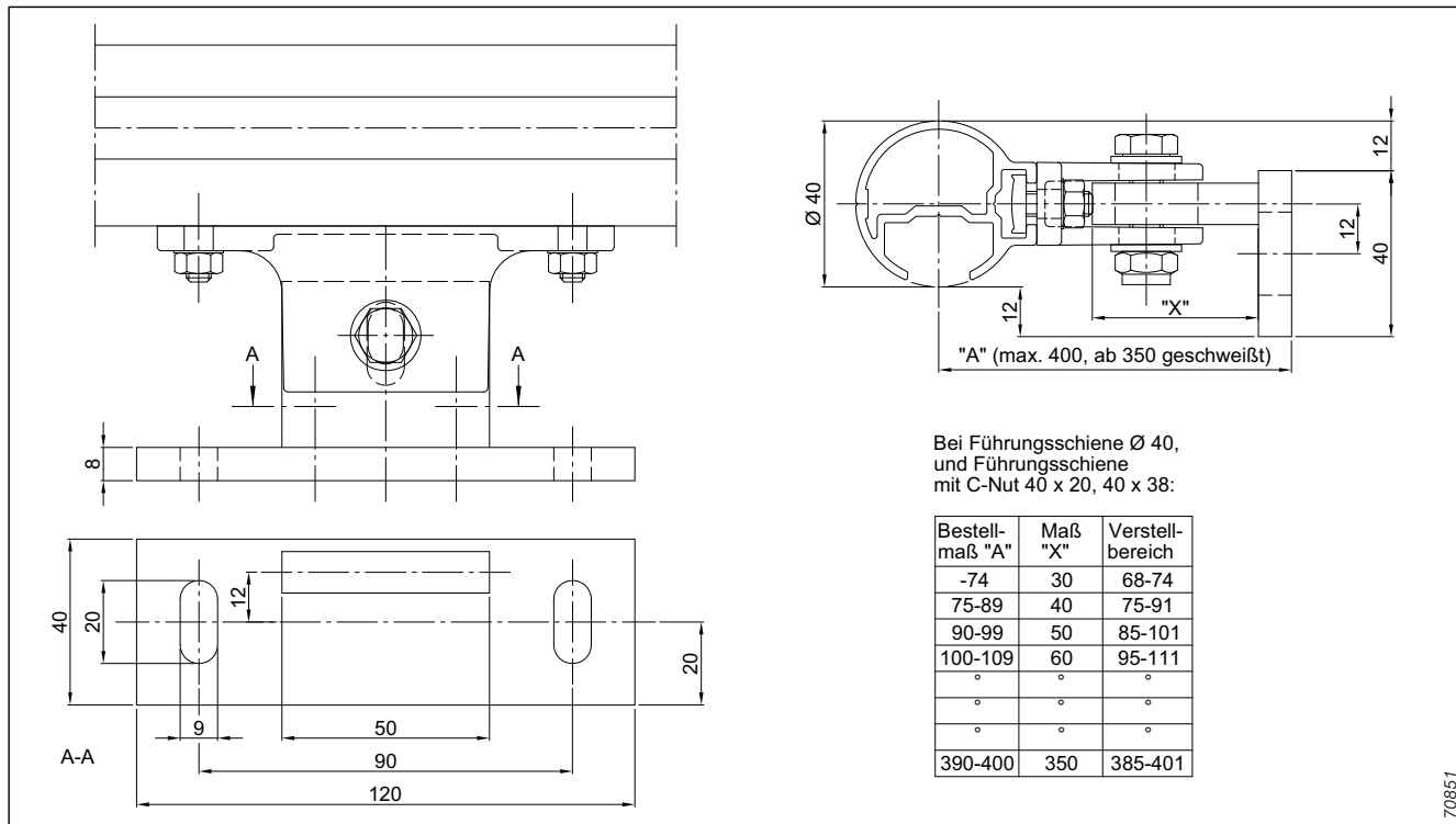
Abb. 199: Führungsschienenhalter Nr. H115
