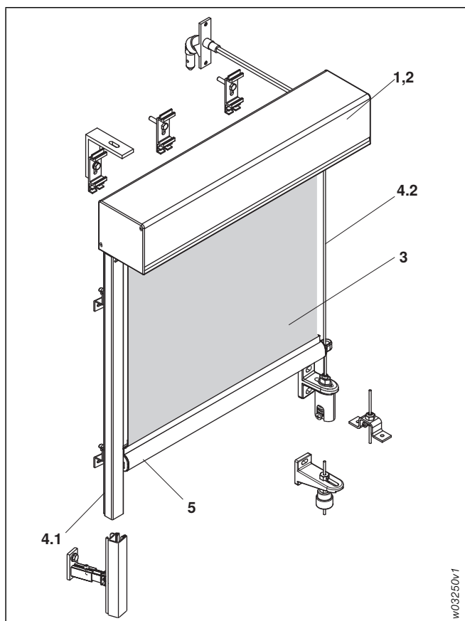
Abb. 26: Senkrecht-Markise 490
