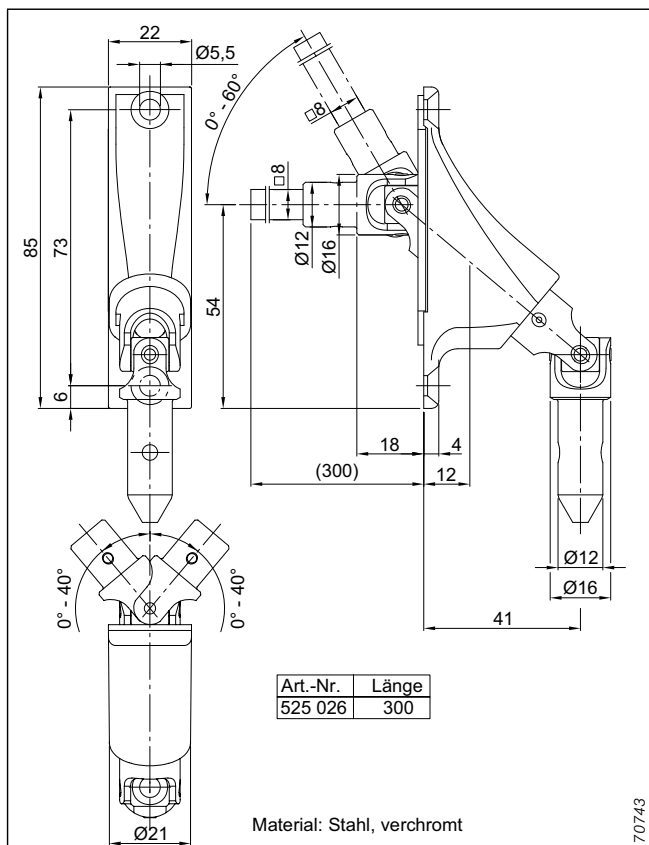
Abb. 193: Gelenkplatte 0°-60°
