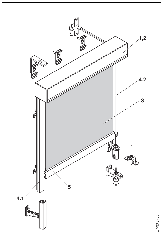
Abb. 1: Senkrecht-Markise 470
