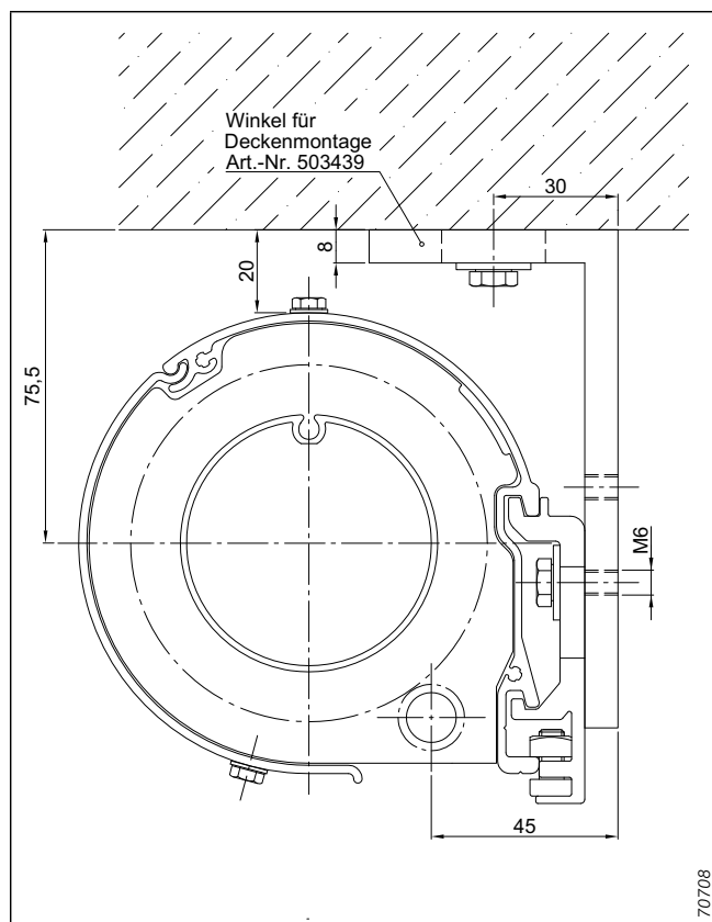
Abb. 84: Deckenmontage Typ 46.3
