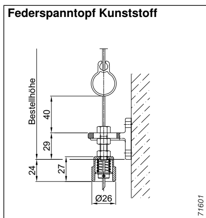
Abb. 7: Federspanntopf Kunststoff
