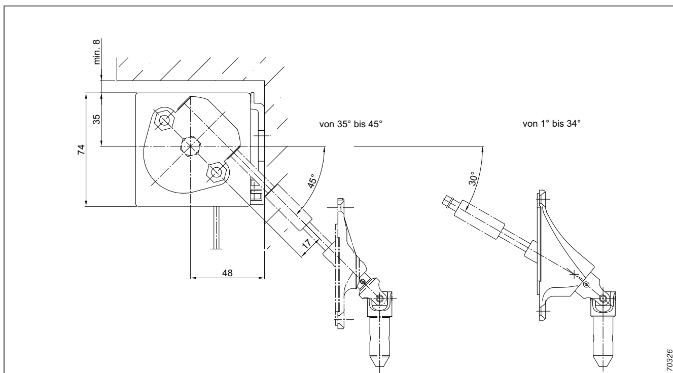
Abb. 14: Getriebeabgang 1–45°
