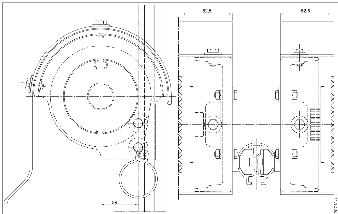
Abb. 180: Fassaden-Markise 201 mit Halbrundblende Typ 2.3 zwischen den Schienen
