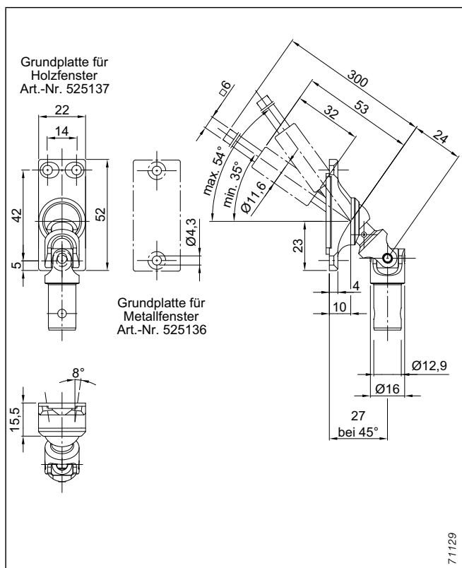
Abb. 237: Gelenkplatte 35°–54°
