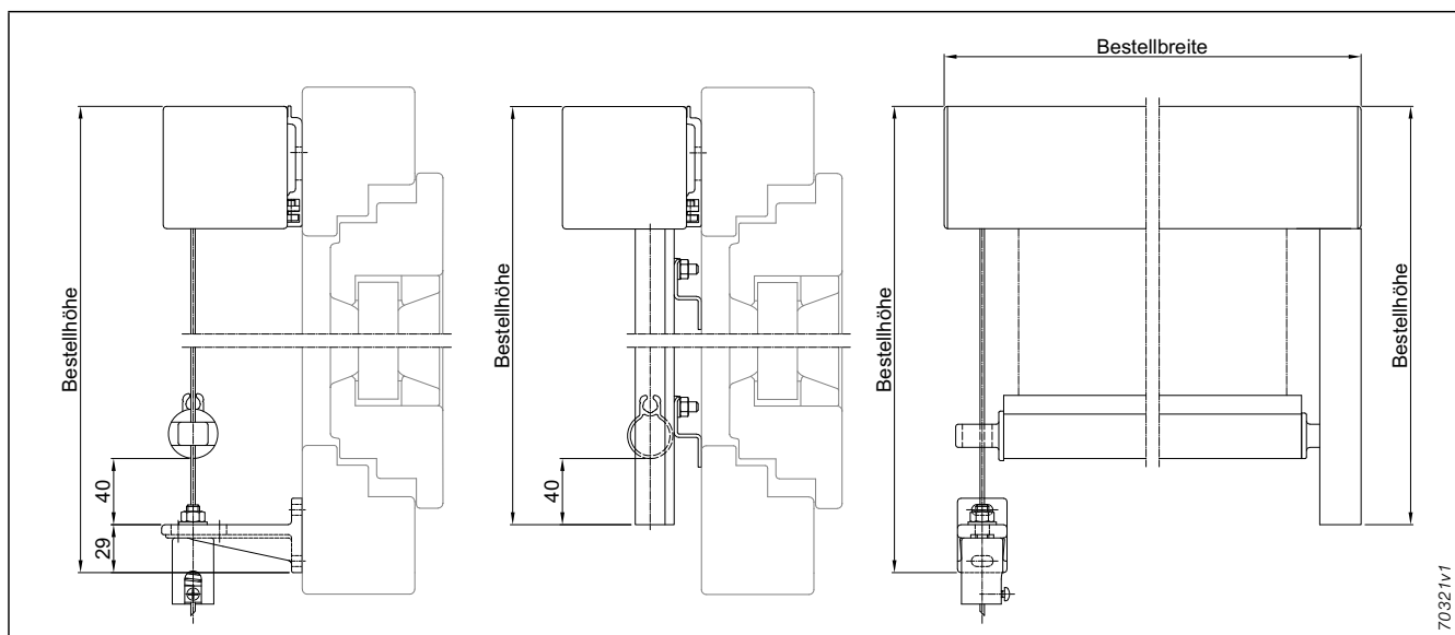
Abb. 3: Maßanleitung
