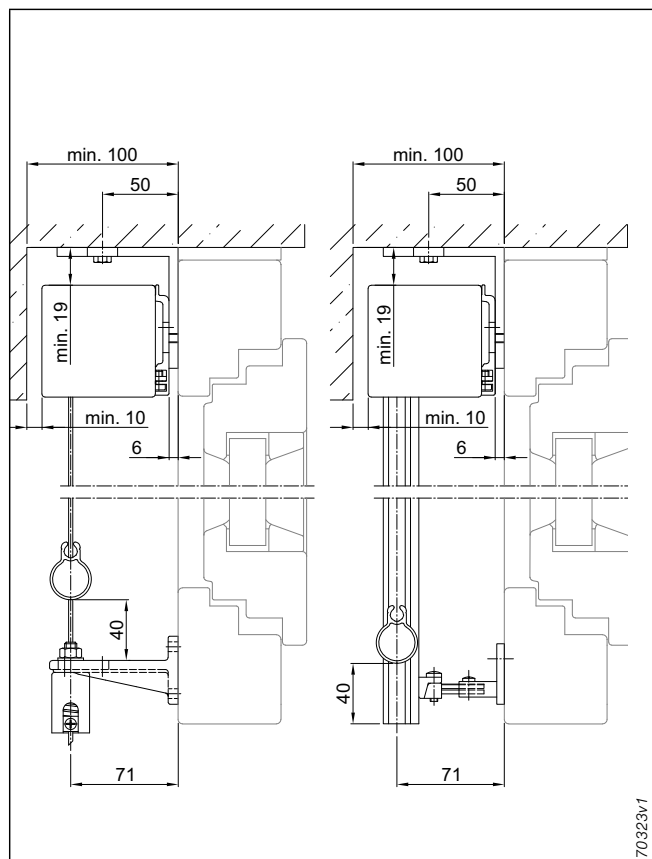
Abb. 12: Senkrecht-Markise 470, Rechtsroller, Deckenmontage
