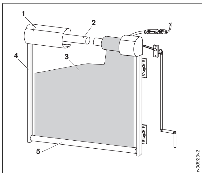
Abb. 217: Fassaden-Markise 209
