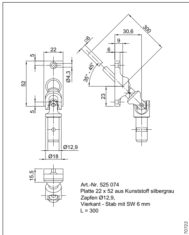
Abb. 104: Gelenkplatte 35°–45° für Kurbelantrieb außen
