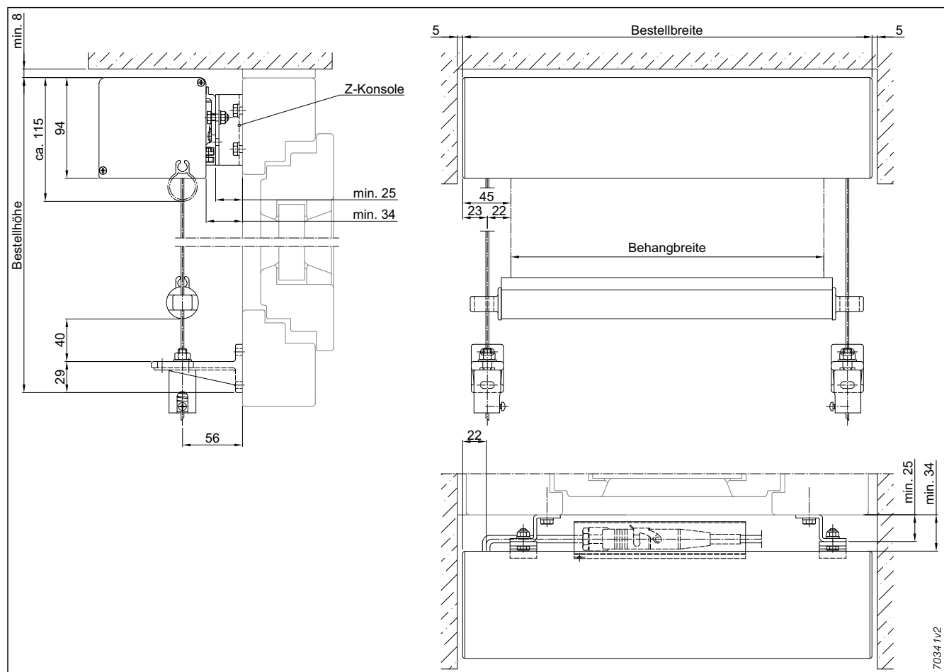
Abb. 41: Einzelanlage, Linksroller, Wandmontage, Seilführung mit Leitungsaustritt hinten
