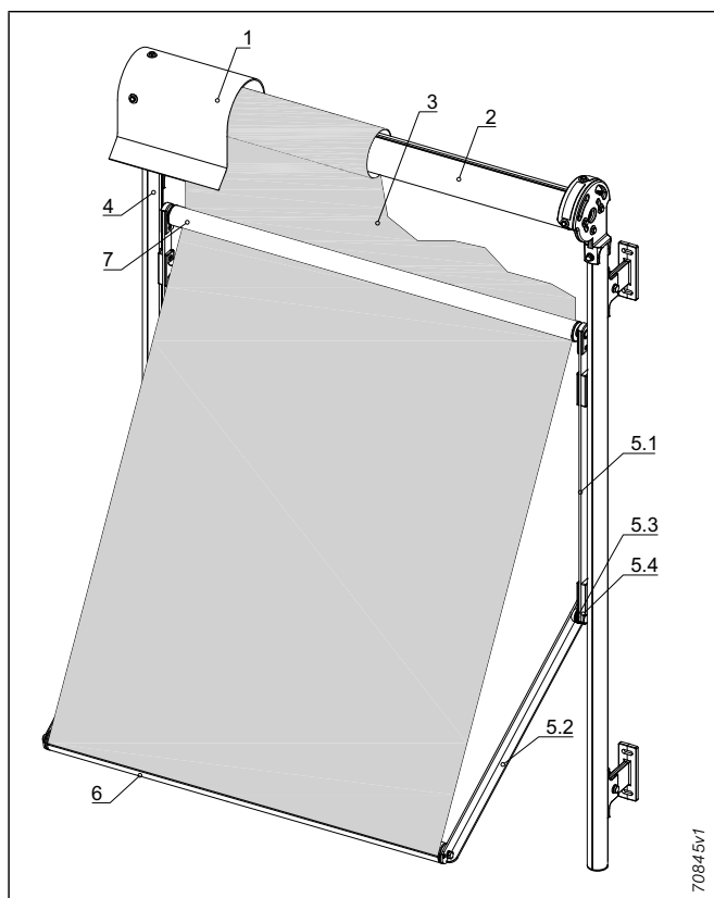
Abb. 240: Markisolette 101
