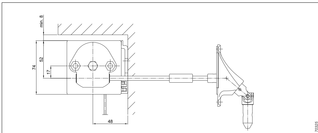
Abb. 13: Getriebeabgang 0°
