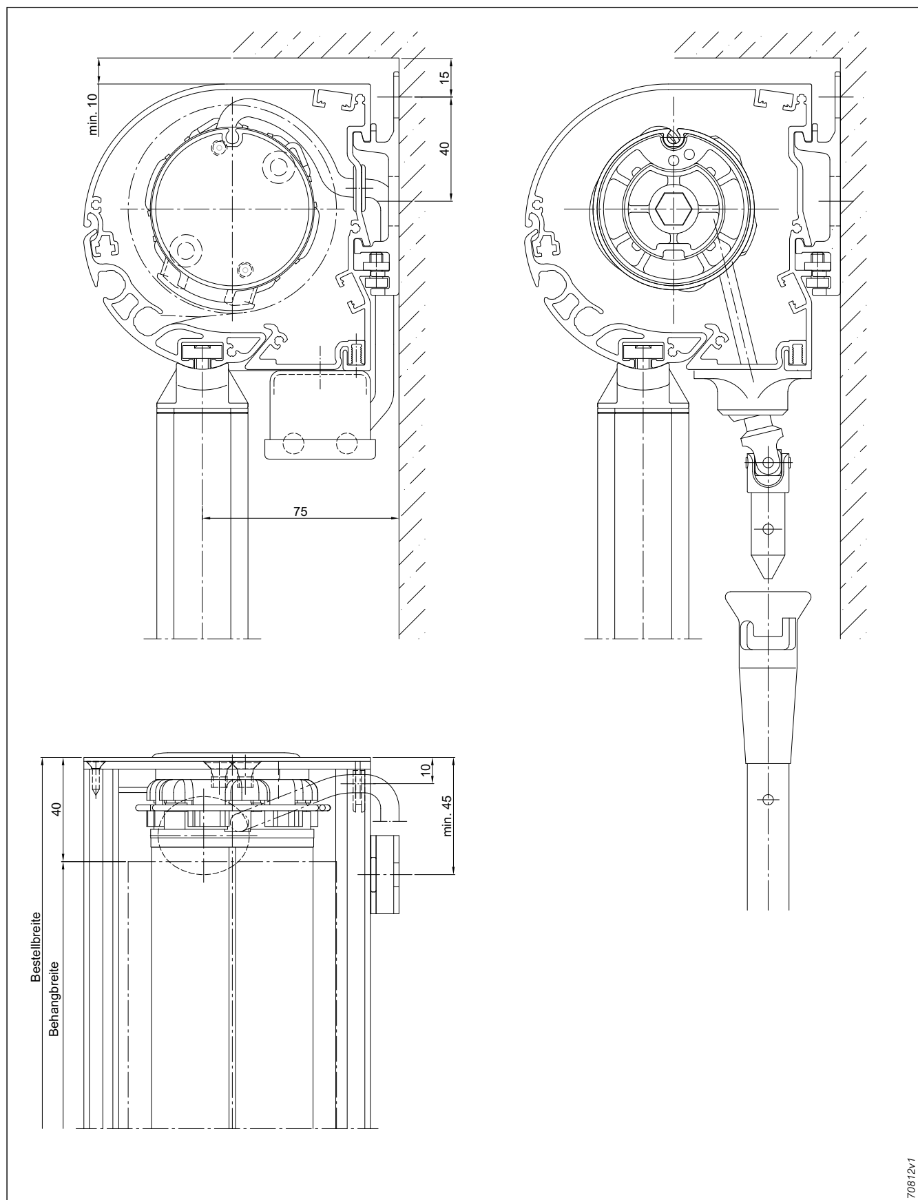
Abb. 132: Fallarm-Markise 355: Motorbedienung und Kurbelbedienung von außen
