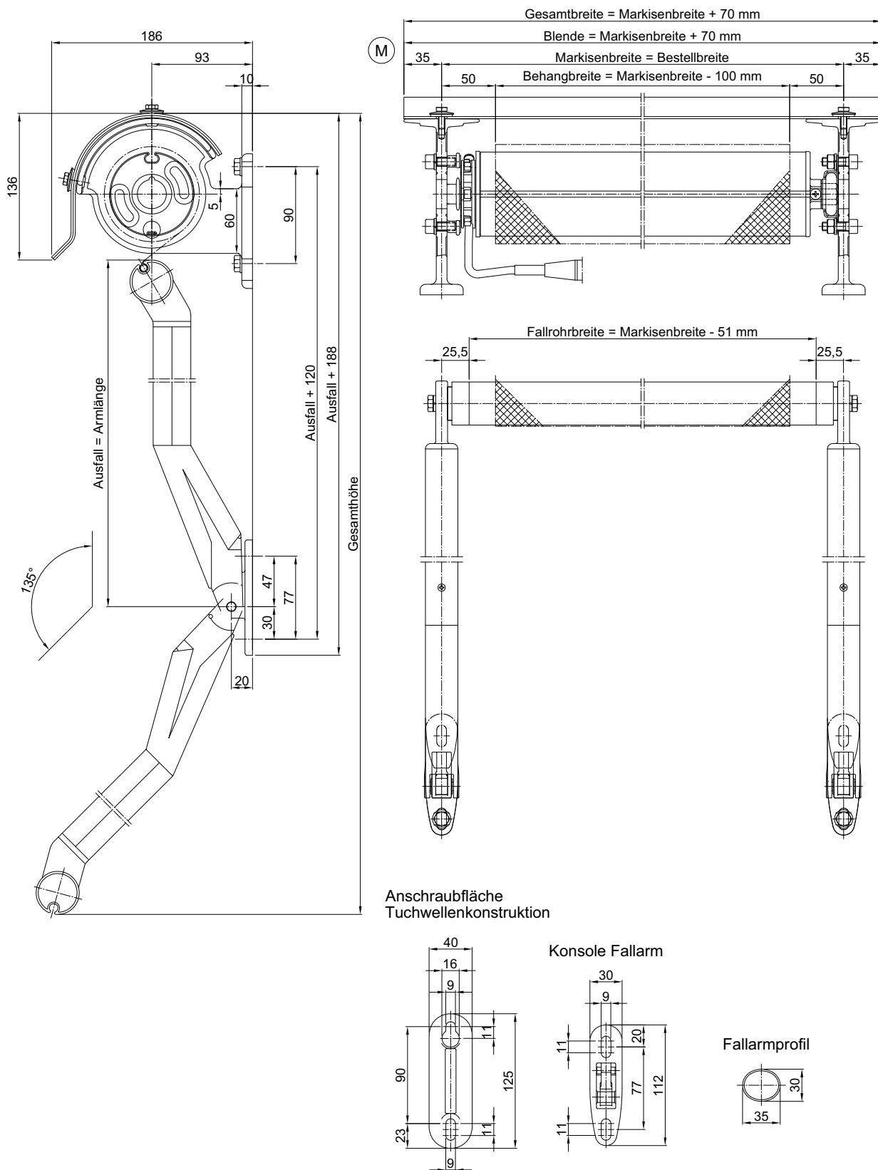
Abb. 137: Maßanleitung Fallarm-Markise 340 (Einzelanlage)
