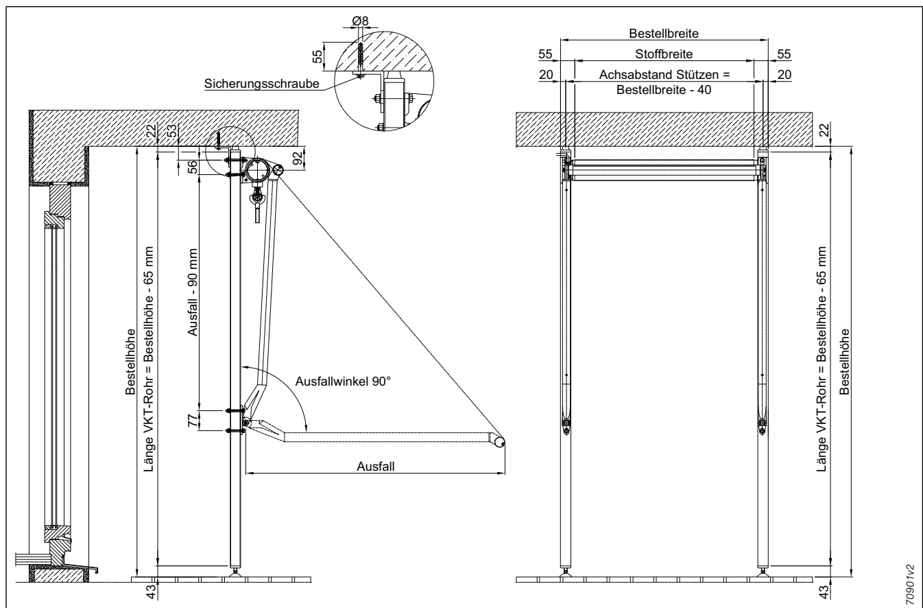
Abb. 159: Montage mit Klemmsttze
