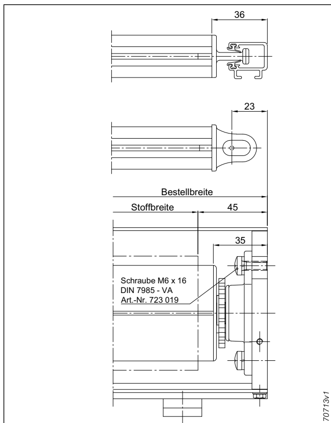
Abb. 78: Spindelsperre
