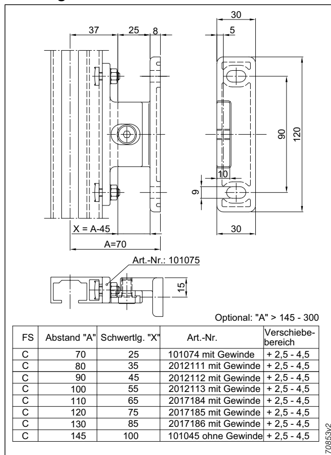
Abb. 201: Führungsschienenhalter Nr. 8
