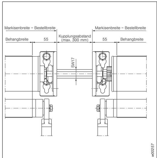
Abb. 158: Kupplungsabstand
