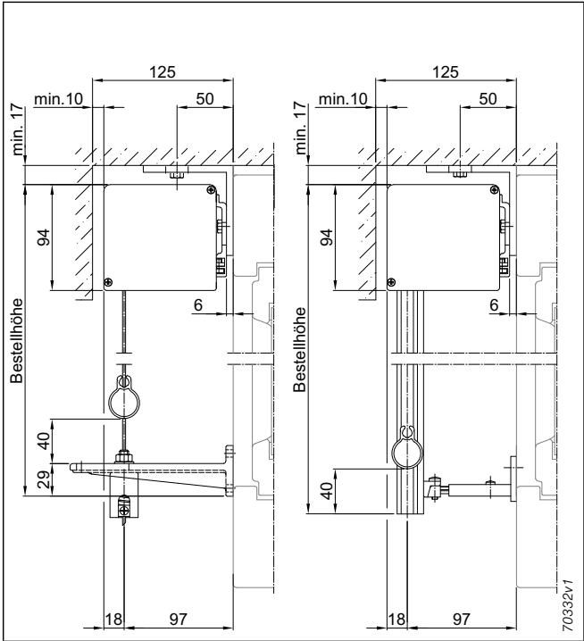
Abb. 37: Senkrecht-Markise 490, Deckenmontage
