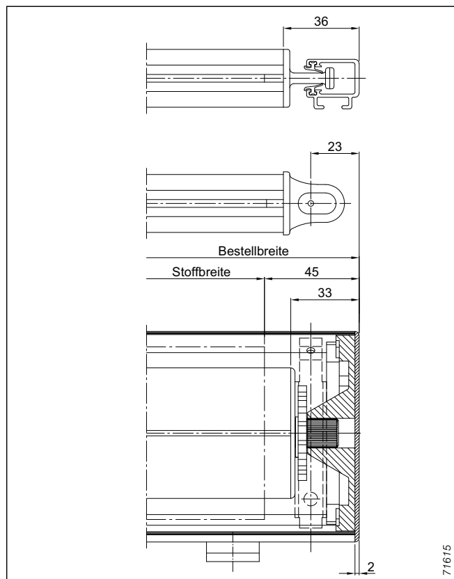
Abb. 52: Spindelsperre
