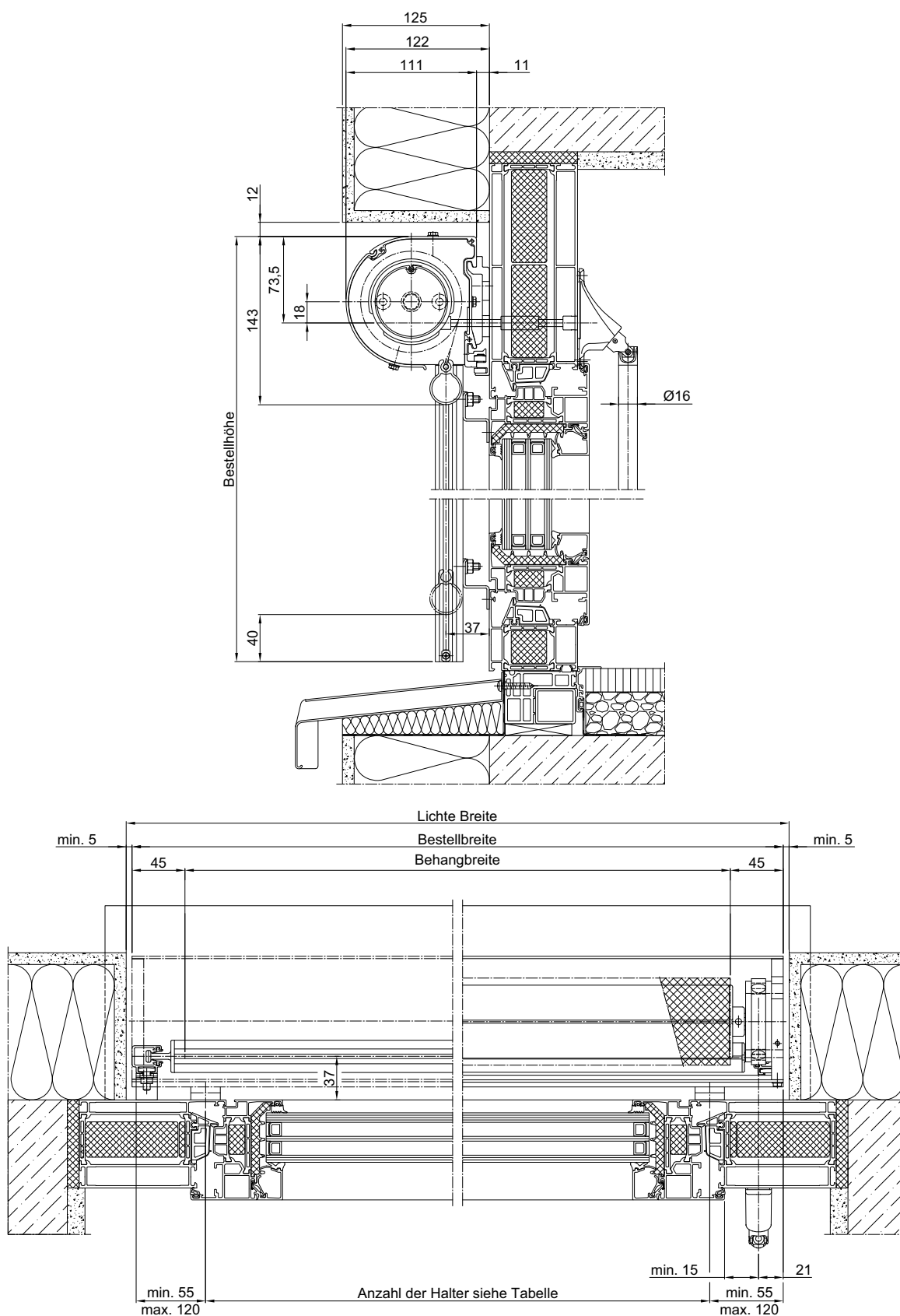
Abb. 72: Senkrecht-Markise 499 – Schienenführung, Kurbelantrieb
