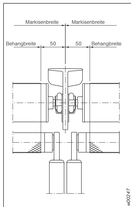
Abb. 147: Endlager – Endlager
