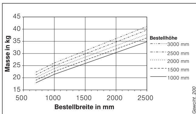
Abb. 166: Gewicht Typ 200
