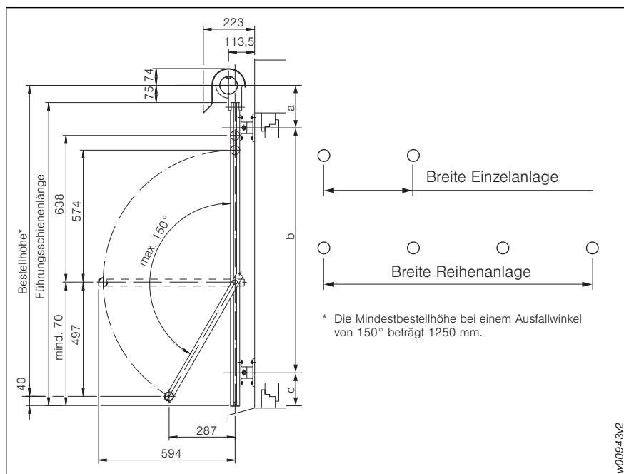
Abb. 244: Maßanleitung Markisolette 101
