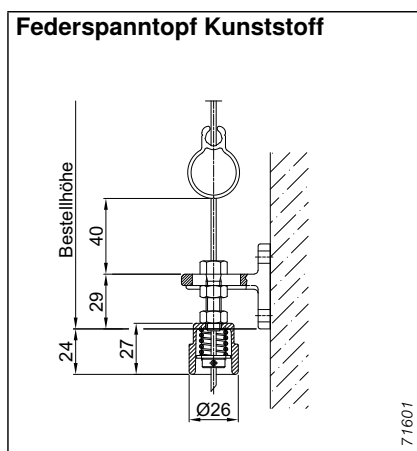
Abb. 32: Federspanntopf Kunststoff
