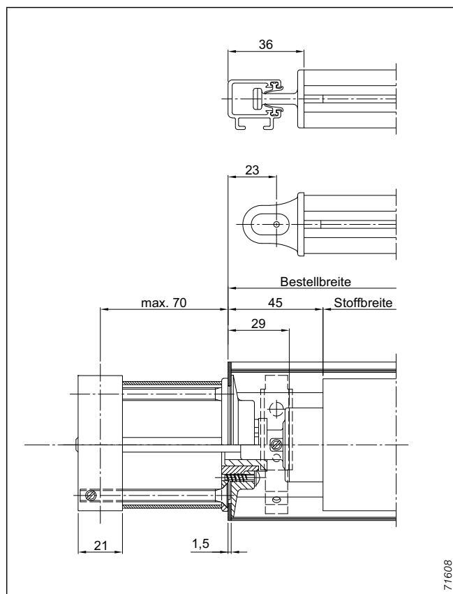
Abb. 22: Getriebe außenliegend, Standard
