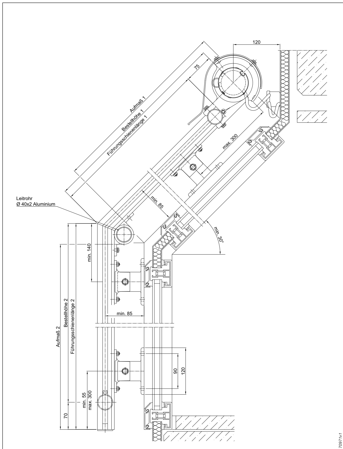
Abb. 179: Fassaden-Markise 203 mit Halbrundblende Typ 2.3 um 40° gedreht
