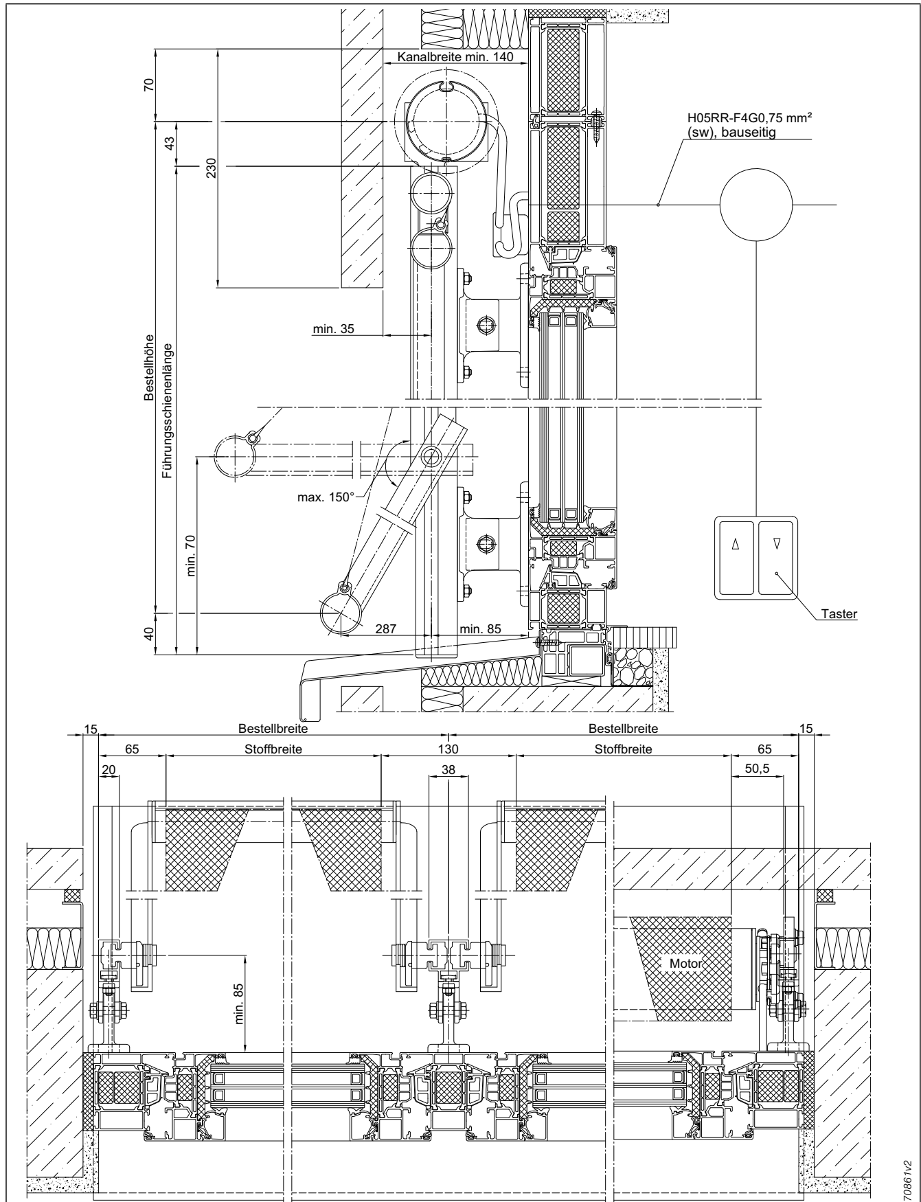
Abb. 249: Markisolette 101, in bauseitigem Kanal, Führungsschiene mit C-Nut 20x40 mm oder 38x40 mm
