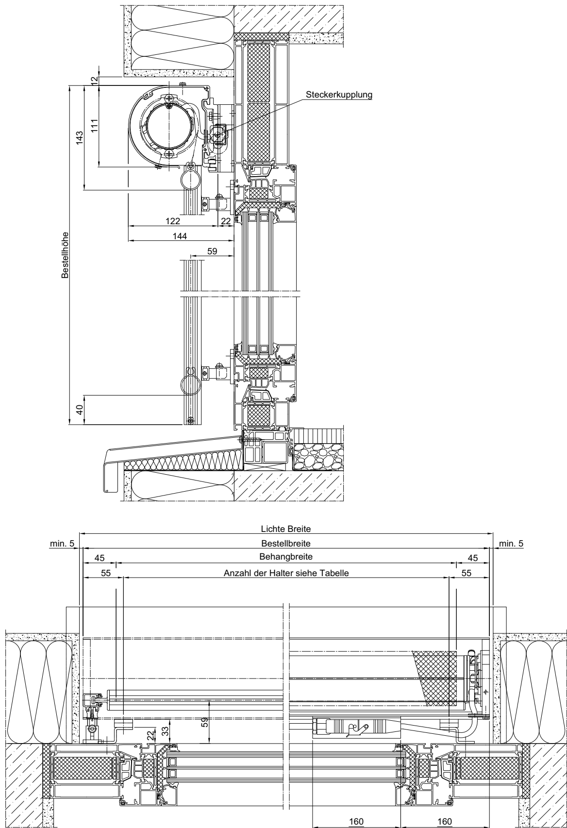
Abb. 74: Senkrecht-Markise 499 – Schienenführung, Motorantrieb
