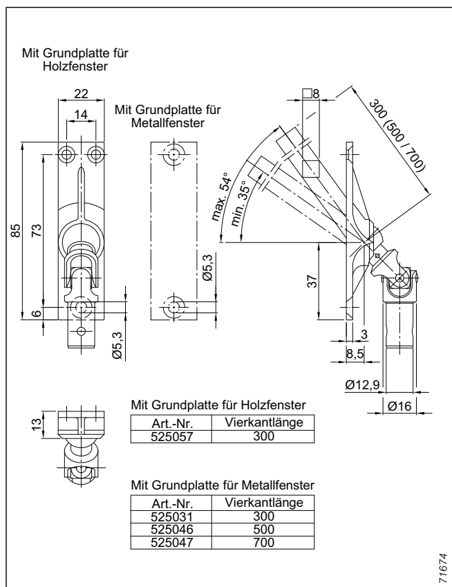
Abb. 190: Gelenkplatte 35°-54°
