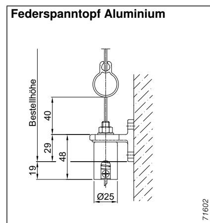
Abb. 122: Federspanntopf Aluminium
